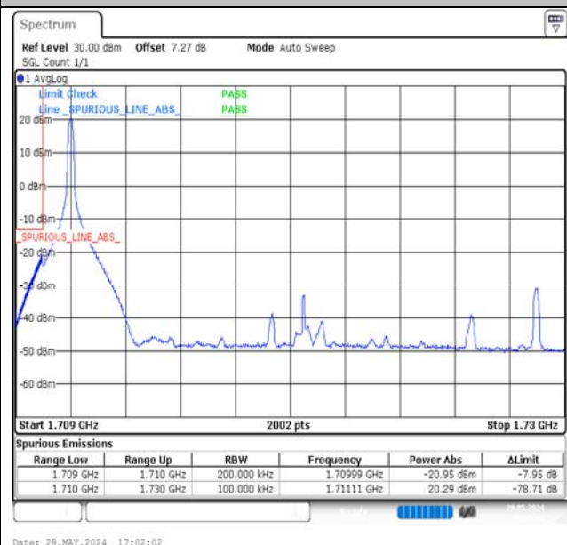
Band66-20MHz-QPSK-132072-1RB#0-PASS
