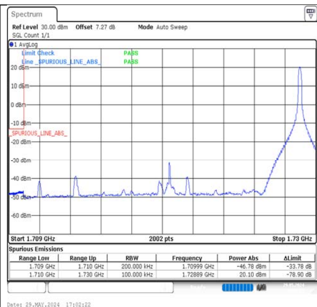
Band66-20MHz-QPSK-132072-1RB#99-PASS
