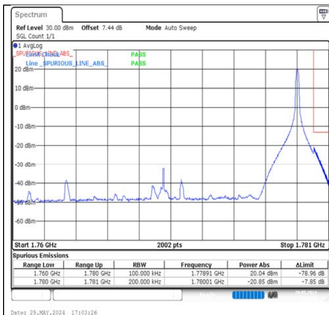
Band66-20MHz-QPSK-132572-1RB#99-PASS
