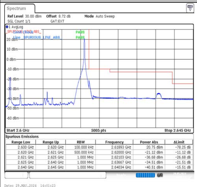
Band38-20MHz-QPSK-38150-1RB#99-PASS
