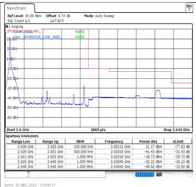
Band38-20MHz-QPSK-38150-1RB#0-PASS
