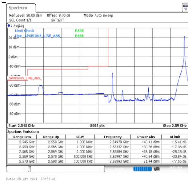
Band38-20MHz-QPSK-37850-1RB#99-PASS
