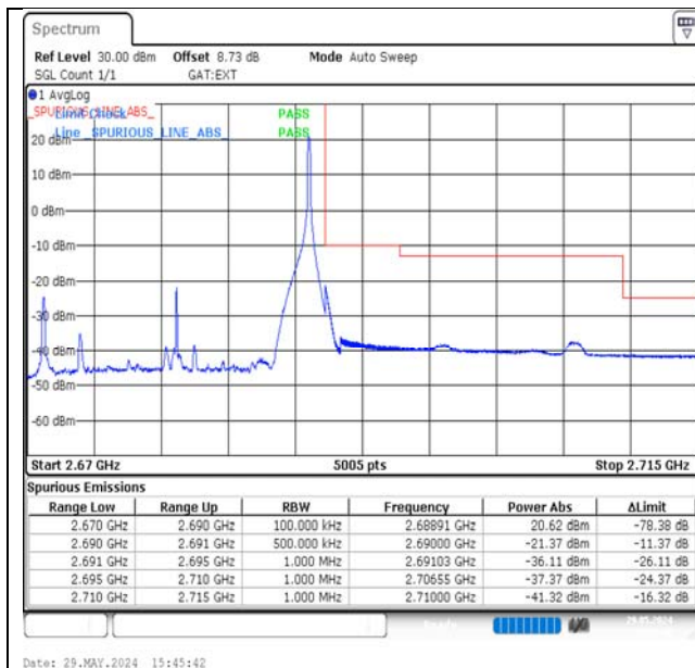
Band41-20MHz-QPSK-41490-1RB#99-PASS
