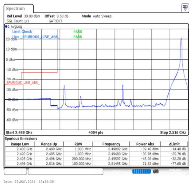
Band41-20MHz-QPSK-39750-1RB#99-PASS
