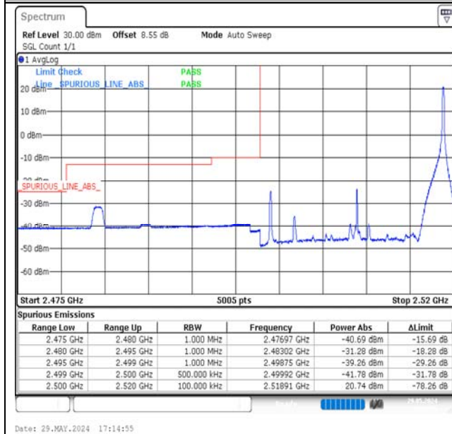
Band7-20MHz-QPSK-20850-1RB#99-PASS
