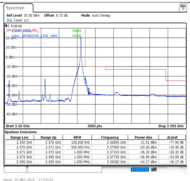
Band7-20MHz-QPSK-21350-1RB#99-PASS
