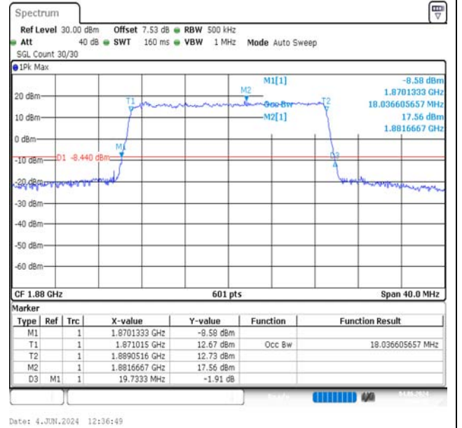
Band2-20MHz-QPSK-18900-100RB#0-PASS
