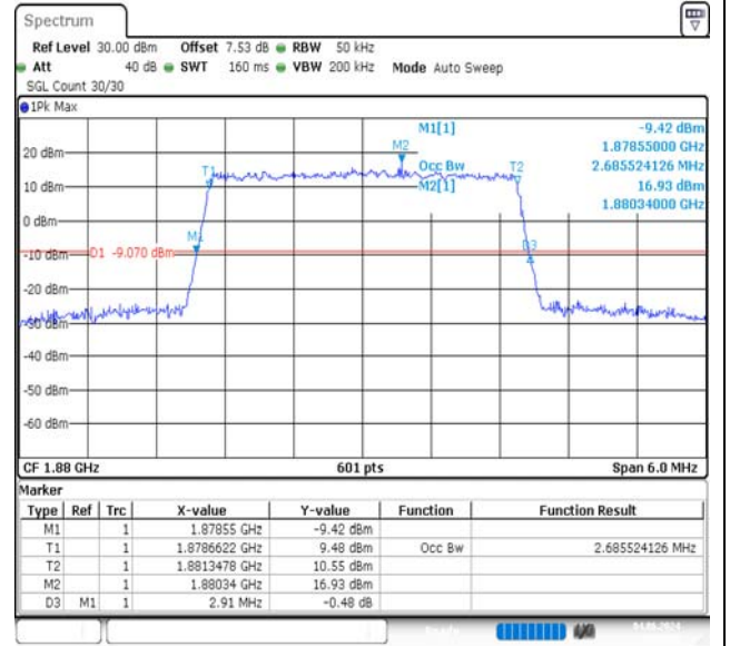
Band2-3MHz-QPSK-18900-15RB#0-PASS
