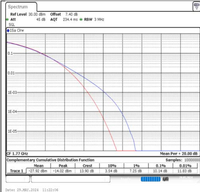
Band66-20MHz-QPSK-132572-1RB#0-PASS
