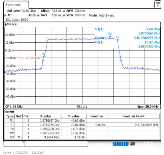
Band2-10MHz-QPSK-18900-50RB#0-PASS
