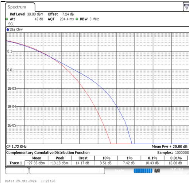
Band66-20MHz-QPSK-132072-1RB#0-PASS
