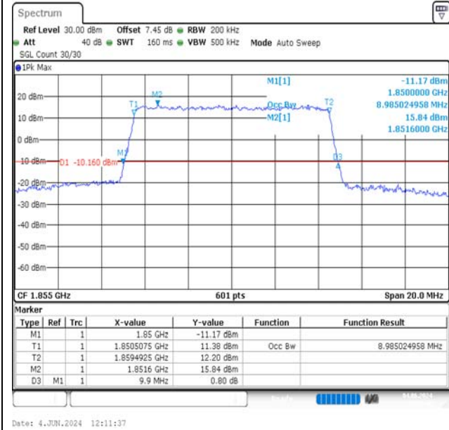
Band2-10MHz-QPSK-18650-50RB#0-PASS
