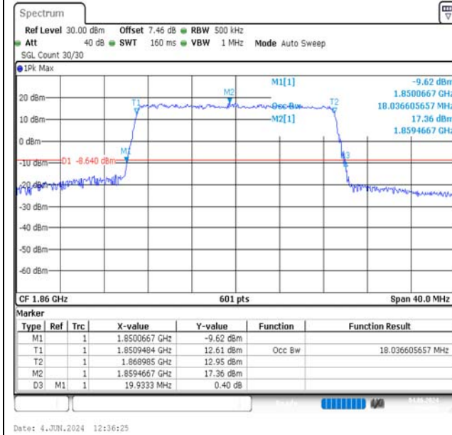
Band2-20MHz-QPSK-18700-100RB#0-PASS
