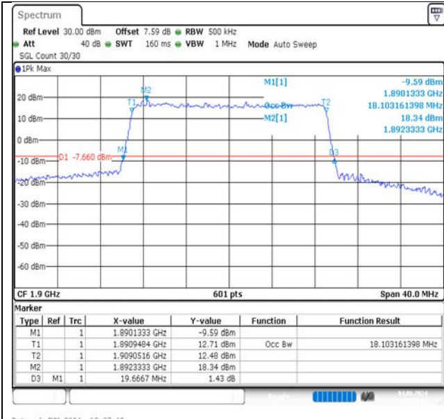
Band2-20MHz-QPSK-19100-100RB#0-PASS
