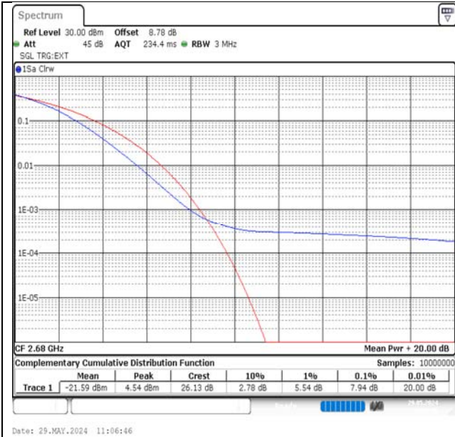
Band41-20MHz-QPSK-41490-1RB#0-PASS
