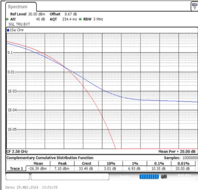
Band38-20MHz-QPSK-37850-1RB#0-PASS
