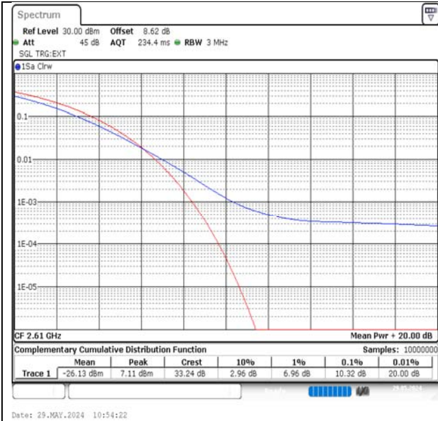
Band38-20MHz-QPSK-38150-1RB#0-PASS
