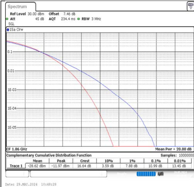
Band2-20MHz-QPSK-18700-1RB#0-PASS
