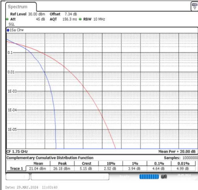
Band4-10MHz-QPSK-20350-1RB#0-PASS
