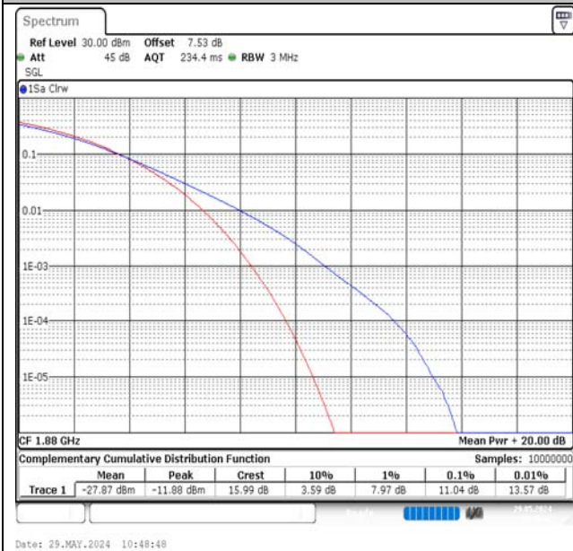
Band2-20MHz-QPSK-18900-1RB#0-PASS
