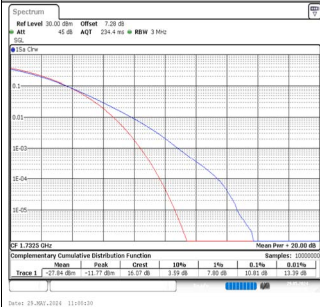
Band4-20MHz-QPSK-20175-1RB#0-PASS
