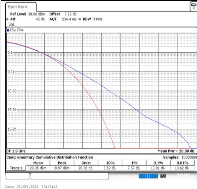
Band2-20MHz-16QAM-19100-1RB#0-PASS
