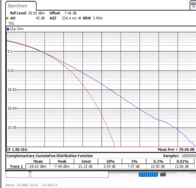
Band2-20MHz-16QAM-18700-1RB#0-PASS
