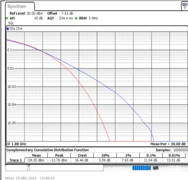
Band2-20MHz-16QAM-18900-1RB#0-PASS
