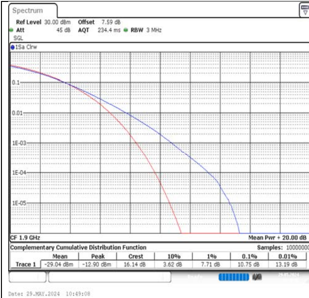
Band2-20MHz-QPSK-19100-1RB#0-PASS
