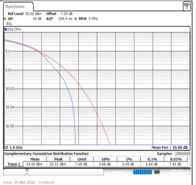
Band2-20MHz-QPSK-19100-100RB#0-PASS
