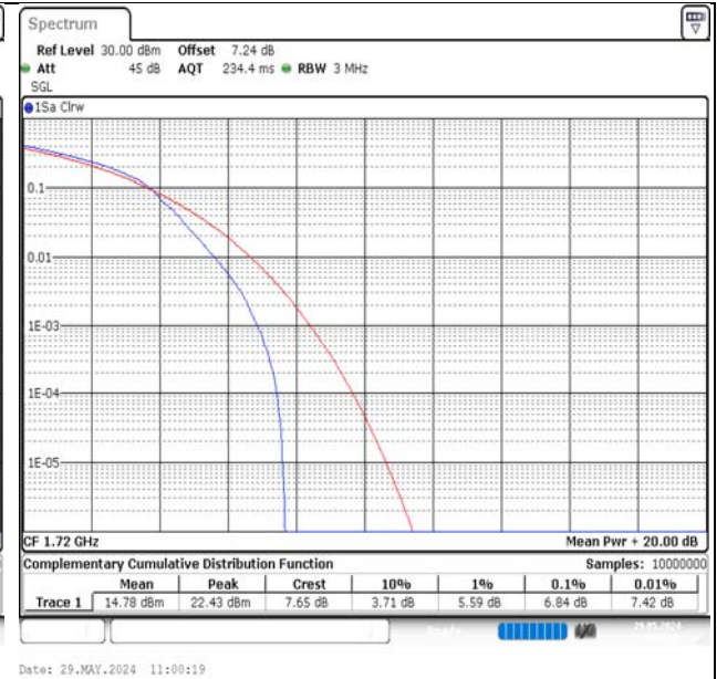
Band4-20MHz-QPSK-20050-100RB#0-PASS
