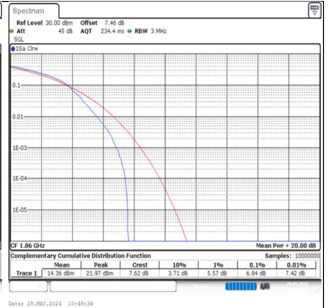
Band2-20MHz-QPSK-18700-100RB#0-PASS
