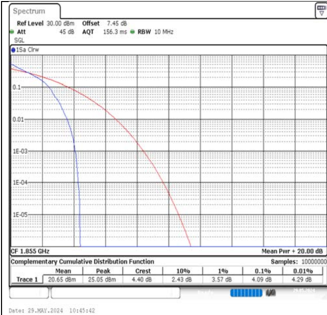
Band2-10MHz-QPSK-18650-1RB#0-PASS
