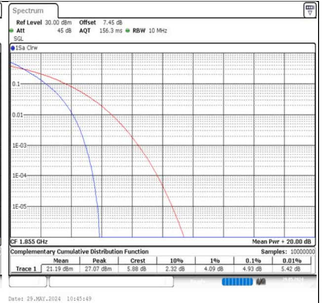
Band2-10MHz-QPSK-18650-50RB#0-PASS
