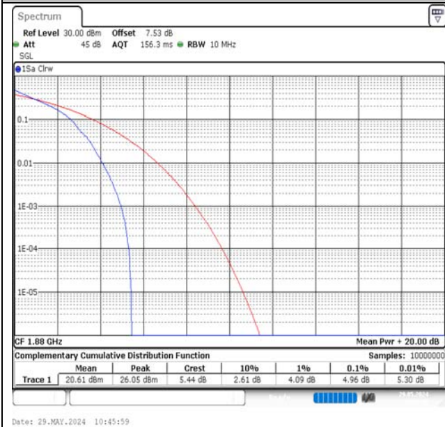
Band2-10MHz-QPSK-18900-1RB#0-PASS
