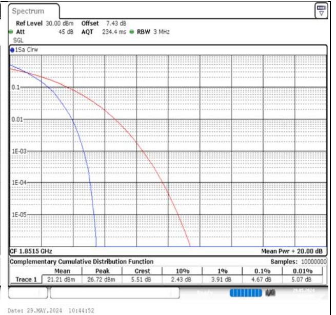
Band2-3MHz-QPSK-18615-15RB#0-PASS
