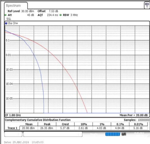
Band2-3MHz-QPSK-18900-1RB#0-PASS
