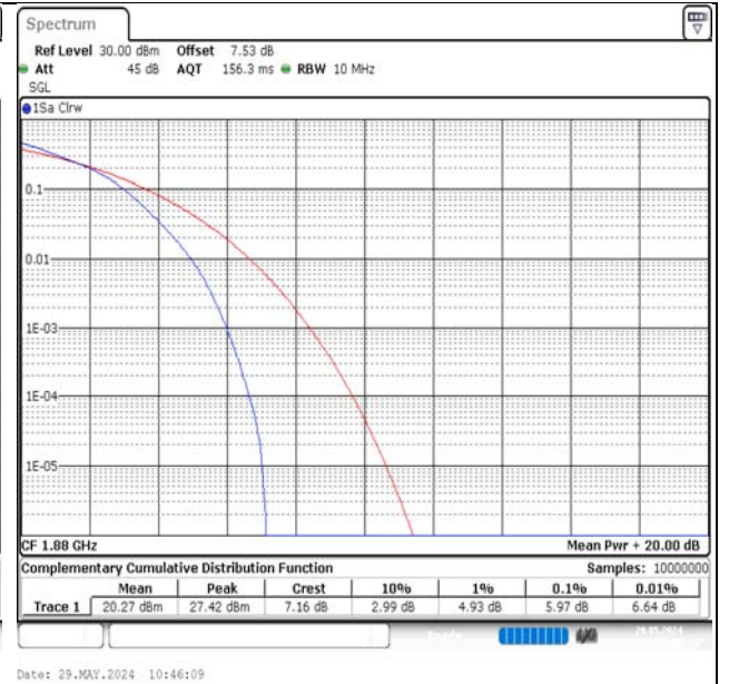
Band2-10MHz-16QAM-18900-50RB#0-PASS
