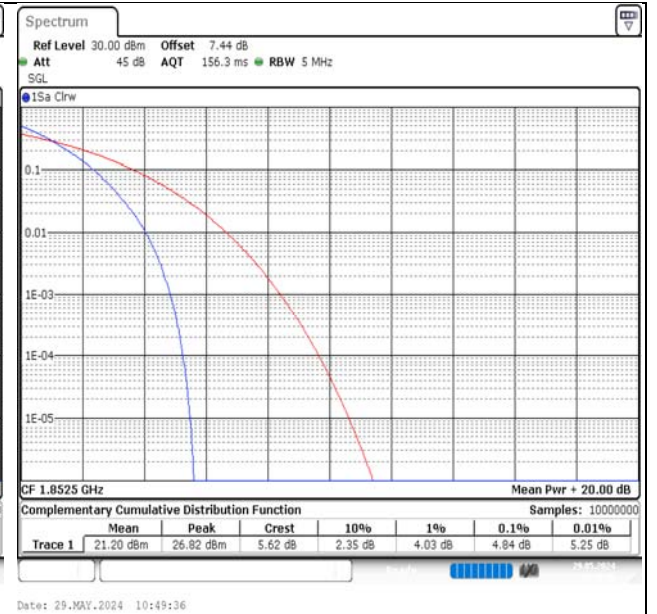
Band2-5MHz-QPSK-18625-25RB#0-PASS
