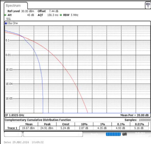
Band2-5MHz-16QAM-18625-1RB#0-PASS
