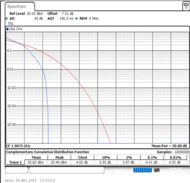
Band2-5MHz-QPSK-19175-1RB#0-PASS
