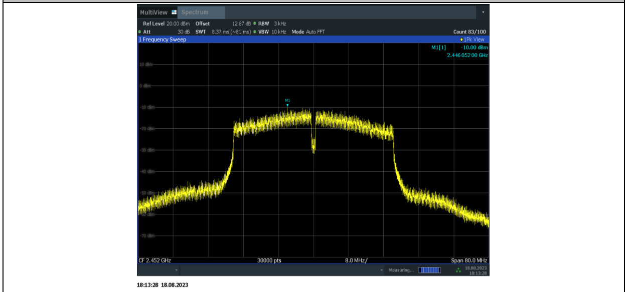
11N40_Ant1_2452
