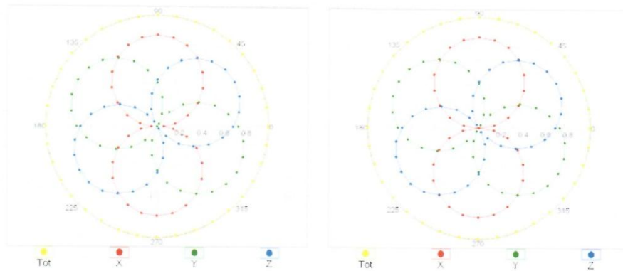
f=1800 MHz,R22
