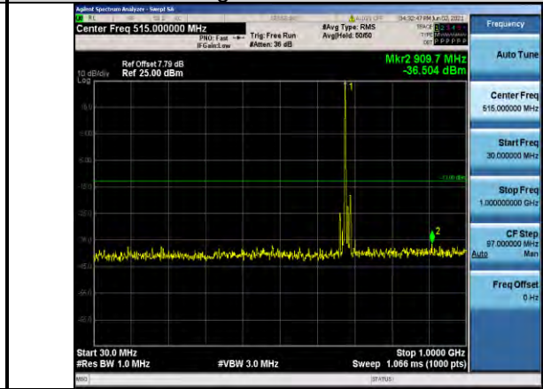
Band71-15MHz-QPSK-133397-1RB#0-Range1:30~1000MHz
