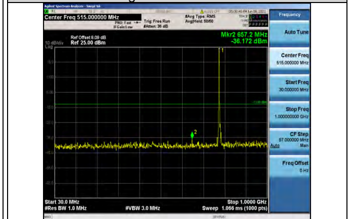
Band13-5MHz-QPSK-23230-1RB#0- Range1:30~1000MHz
