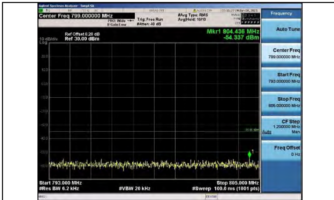
Band13-5MHz-QPSK-23255-1RB#0- Range5:793~805MHz
