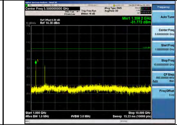
Band71-20MHz-QPSK-133372-1RB#0-Range2:1000~10000MHz
