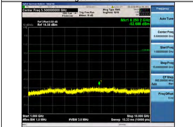
Band13-5MHz-QPSK-23255-1RB#0- Range2:1000~10000MHz
