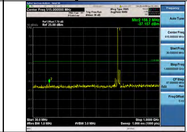
Band71-20MHz-QPSK-133372-1RB#0-Range1:30~1000MHz
