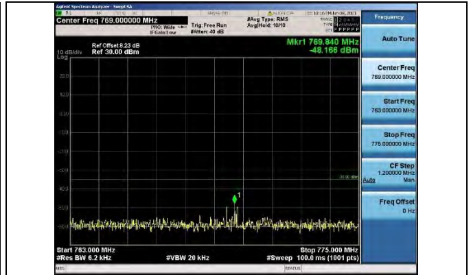
Band13-5MHz-16QAM-23230-1RB#0- Range4: 763~775MHz
