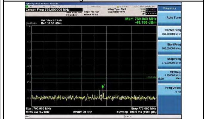
Band 13-5MHz-QPSK-23255-1RB#0-Range4:763~775MHz
