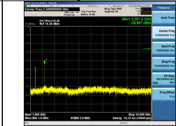
Band71-15MHz-QPSK-133397-1RB#0-Range2:1000~10000MHz
