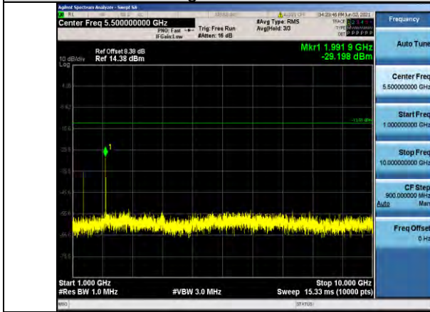
Band71-20MHz-QPSK-133222-1RB#0-Range2:1000~10000MHz
