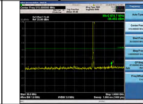
Band71-5MHz-QPSK-133447-1RB#0-Range1:30~1000MHz
