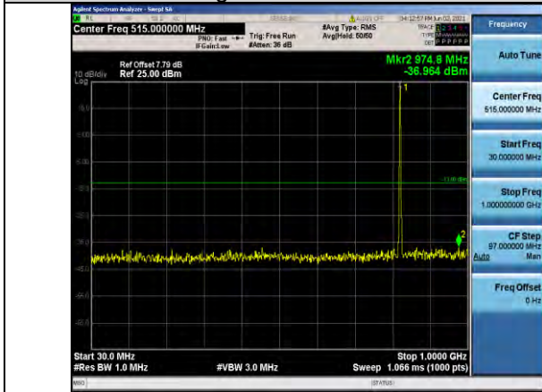
Band5-3MHz-QPSK-20415-1RB#0- Range1:30~1000MHz
