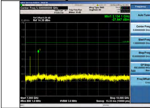
Band12-5MHz-QPSK-23155-1RB#0- Range2:1000~10000MHz
