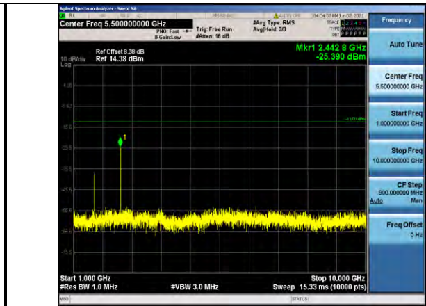
Band26-1.4MHz-QPSK-26697-1RB#0-Range2:1000~10000MHz
