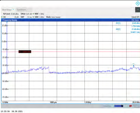
Band66-10MHz-QPSK-132622-1RB#0- Range2:1000~20000MHz
