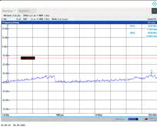
Band66-20MHz-QPSK-132572-1RB#0- Range2:1000~20000MHz
