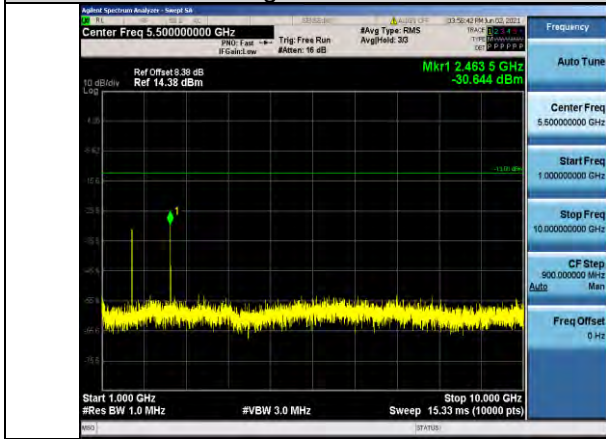
Band26-3MHz-QPSK-26775-1RB#0- Range2:1000~10000MHz
