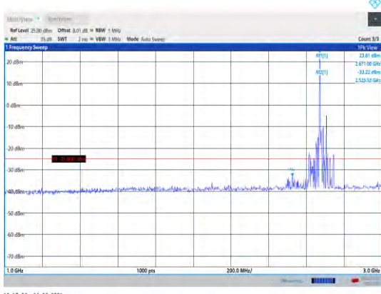
Band41-20MHz-QPSK-41490-1RB#0- Range2:1000~3000MHz
