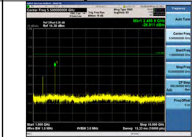
Band5-10MHz-QPSK-20525-1RB#0- Range2:1000~10000MHz
