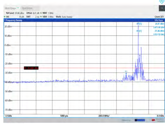
Band41-20MHz-16QAM-41490-1RB#0-Range2:1000~3000MHz
