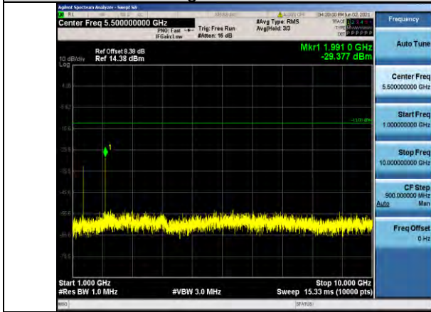
Band71-10MHz-QPSK-133172-1RB#0- Range2:1000~10000MHz
