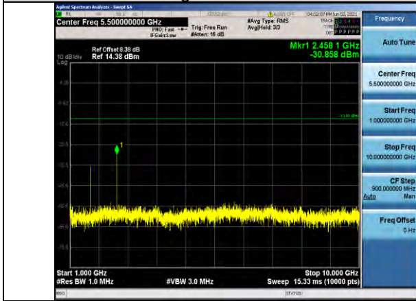
Band26-5MHz-QPSK-26765-1RB#0- Range2:1000~10000MHz
