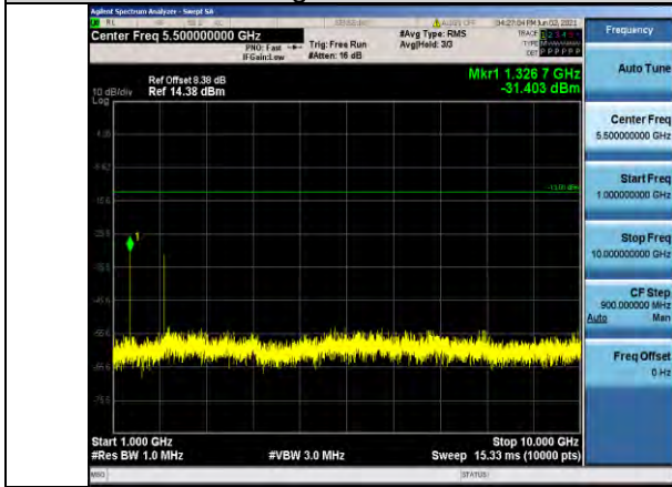
Band71-5MHz-QPSK-133147-1RB#0-Range2:1000~10000MHz
