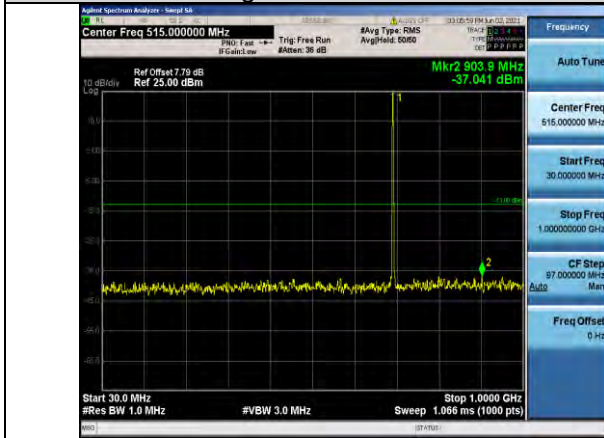
Band12-1.4MHz-QPSK-23017-1RB#0-Range1:30~1000MHz
