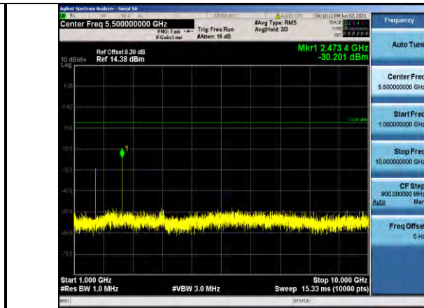
Band5-5MHz-QPSK-20425-1RB#0- Range2:1000~10000MHz
