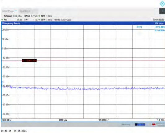
Band66-20MHz-QPSK-132072-1RB#0- Range1:30~1000MHz
