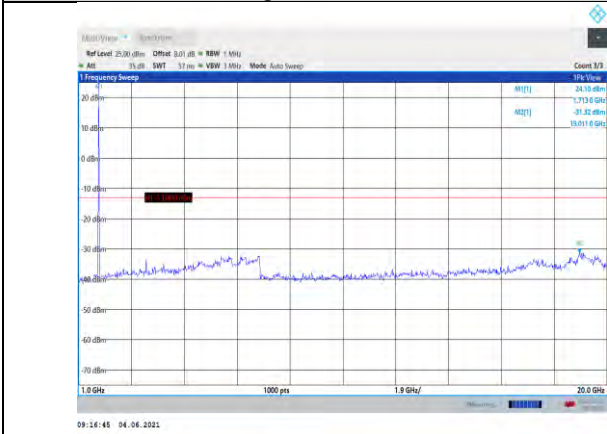
Band4-15MHz-QPSK-20025-1RB#0- Range2:1000~20000MHz
