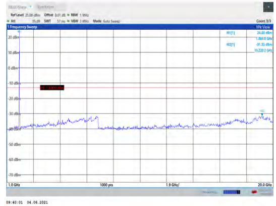
Band25-15MHz-QPSK-26365-1RB#0- Range2:1000~20000MHz
