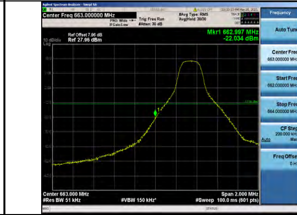
Band71-5MHz-QPSK-133147-1RB#0
