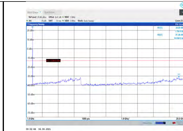
Band4-1.4MHz-QPSK-20175-1RB#0- Range2:1000~20000MHz
