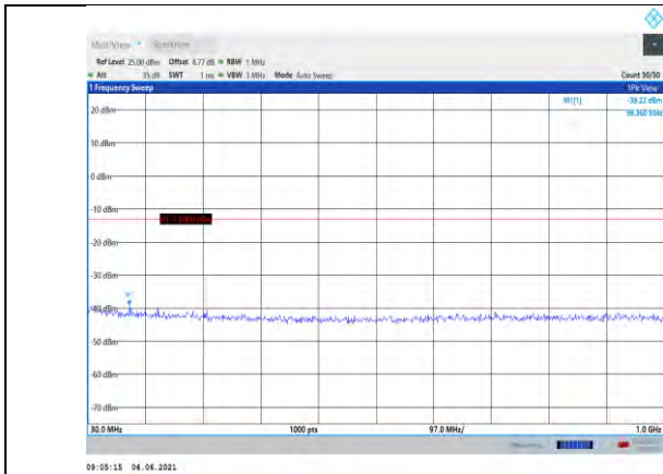
Band4-3MHz-QPSK-19965-1RB#0- Range1:30~1000MHz
