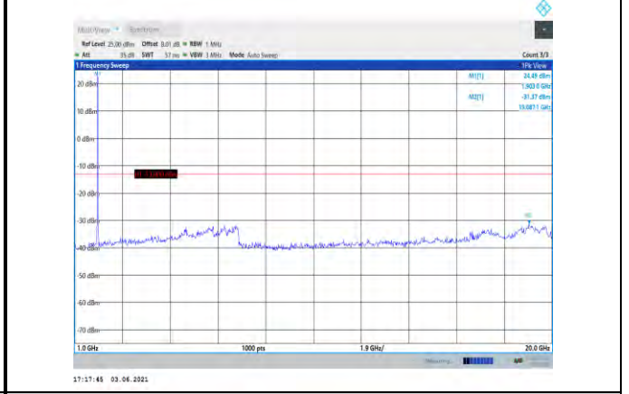
Band2-10MHz-QPSK-19150-1RB#0- Range2:1000~20000MHz
