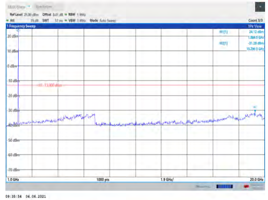
Band25-10MHz-QPSK-26365-1RB#0- Range2:1000~20000MHz
