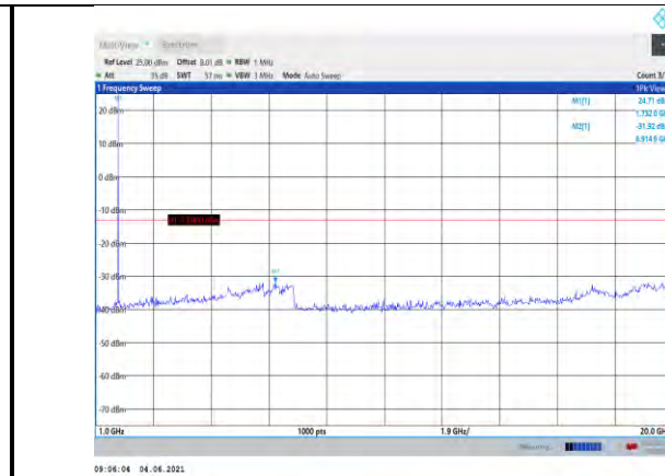
Band4-3MHz-QPSK-20175-1RB#0- Range2:1000~20000MHz
