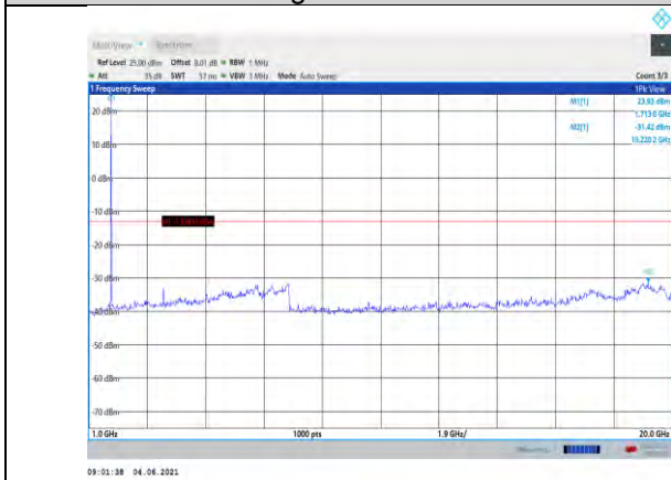
Band4-1.4MHz-QPSK-19957-1RB#0- Range2:1000~20000MHz
