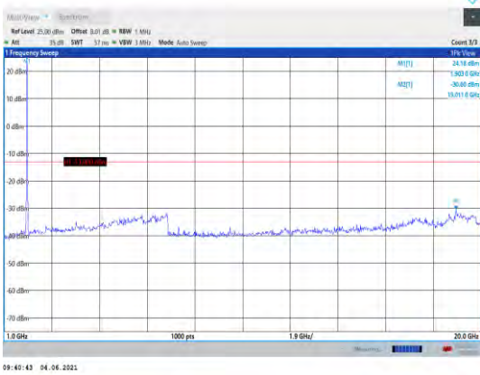
Band25-15MHz-QPSK-26615-1RB#0- Range2:1000~20000MHz
