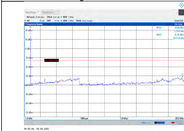
Band4-3MHz-QPSK-19965-1RB#0- Range2:1000~20000MHz
