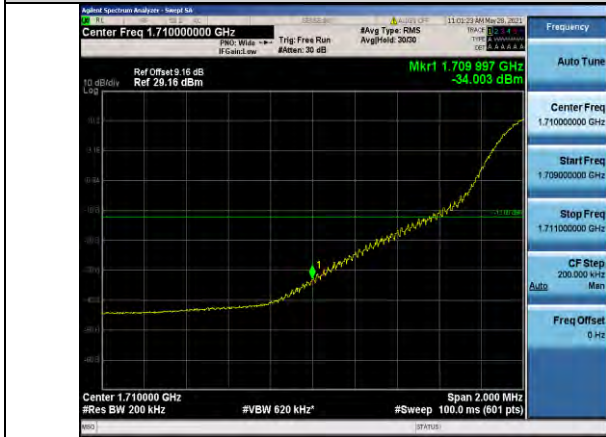
Band66-20MHz-QPSK-132072-1RB#0
