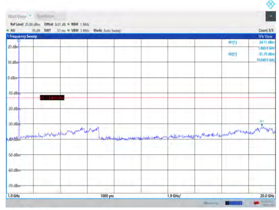
Band25-20MHz-16QAM-26365-1RB#0- Range2:1000~20000MHz
