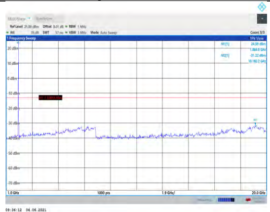
Band25-10MHz-16QAM-26365-1RB#0- Range2:1000~20000MHz
