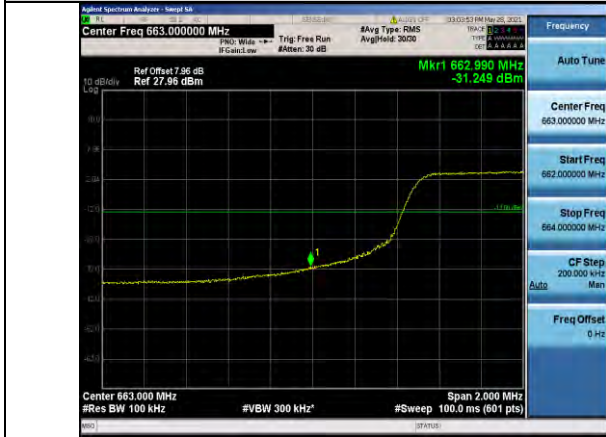
Band71-10MHz-QPSK-133172-50RB#0
