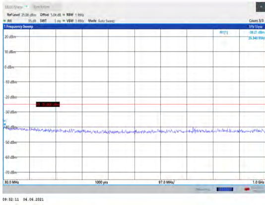
Band41-10MHz-QPSK-39700-1RB#0- Range1:30~1000MHz
