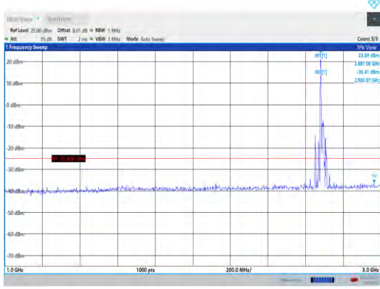
Band41-10MHz-QPSK-41540-1RB#0- Range2:1000~3000MHz
