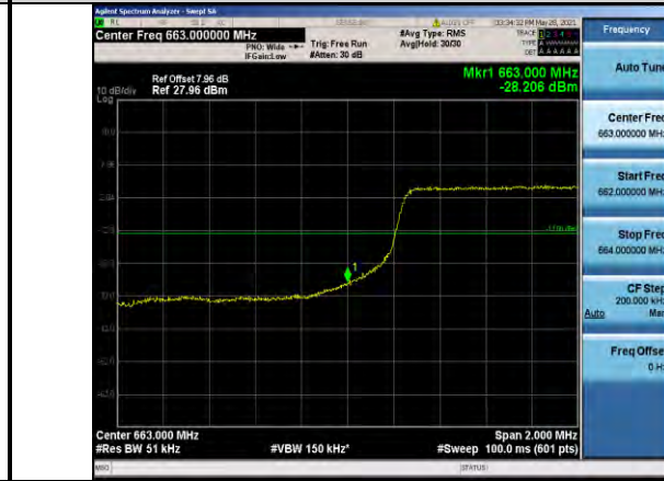
Band71-5MHz-QPSK-133147-25RB#0
