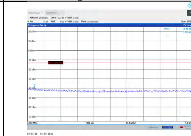
Band4-1.4MHz-QPSK-20393-1RB#0- Range1:30~1000MHz
