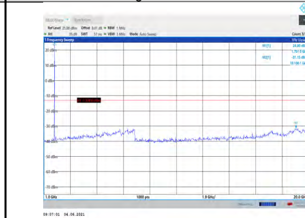
Band4-3MHz-QPSK-20385-1RB#0- Range2:1000~20000MHz
