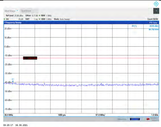
Band25-1.4MHz-QPSK-26365-1RB#0- Range1:30~1000MHz
