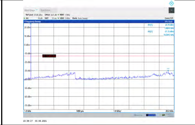
Band2-5MHz-16QAM-19175-1RB#0- Range2:1000~20000MHz
