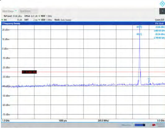
Band41-5MHz-QPSK-41565-1RB#0- Range2:1000~3000MHz
