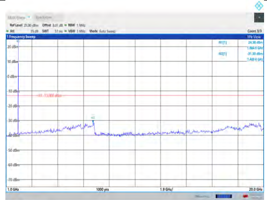
Band25-1.4MHz-QPSK-26365-1RB#0- Range2:1000~20000MHz
