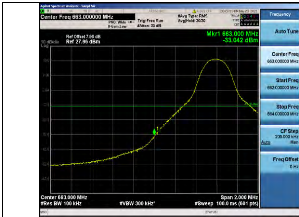
Band71-10MHz-QPSK-133172-1RB#0
