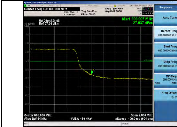
Band71-5MHz-QPSK-133447-25RB#0
