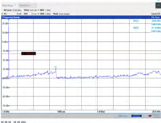
Band25-15MHz-QPSK-26115-1RB#0- Range2:1000~20000MHz
