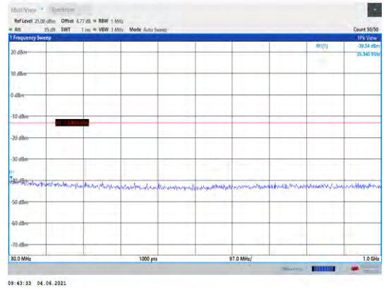
Band25-20MHz-QPSK-26365-1RB#0- Range1:30~1000MHz
