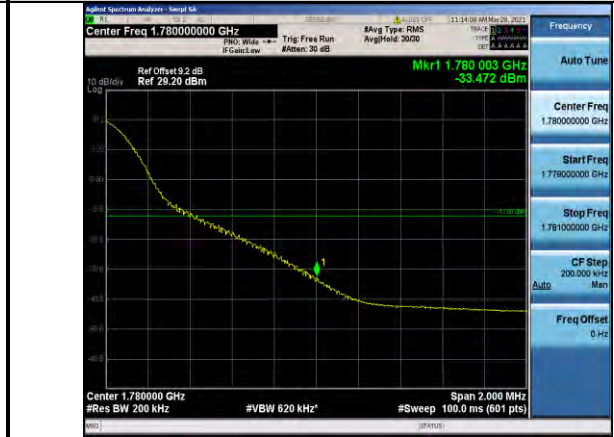
Band66-20MHz-QPSK-132572-1RB#99
