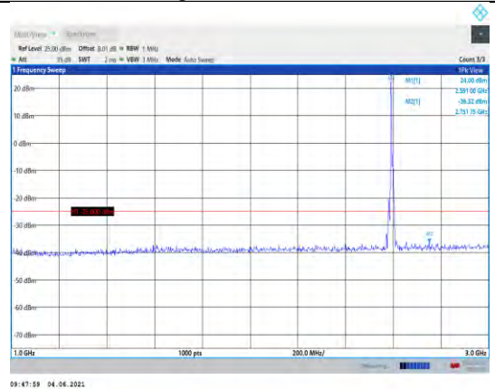
Band41-5MHz-QPSK-40620-1RB#0- Range2:1000~3000MHz
