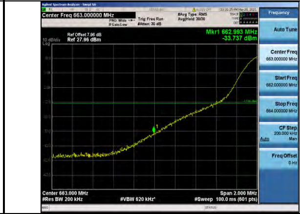
Band71-20MHz-QPSK-133222-1RB#0
