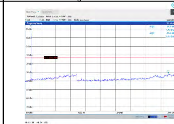
Band4-1.4MHz-QPSK-20393-1RB#0- Range2:1000~20000MHz
