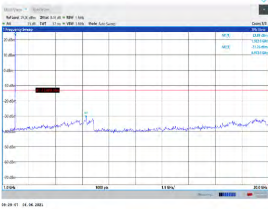
Band25-3MHz-QPSK-26675-1RB#0- Range2:1000~20000MHz
