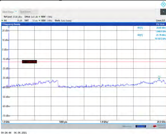
Band25-1.4MHz-QPSK-26047-1RB#0- Range2:1000~20000MHz
