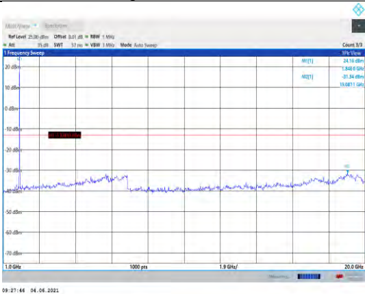
Band25-3MHz-QPSK-26055-1RB#0- Range2:1000~20000MHz
