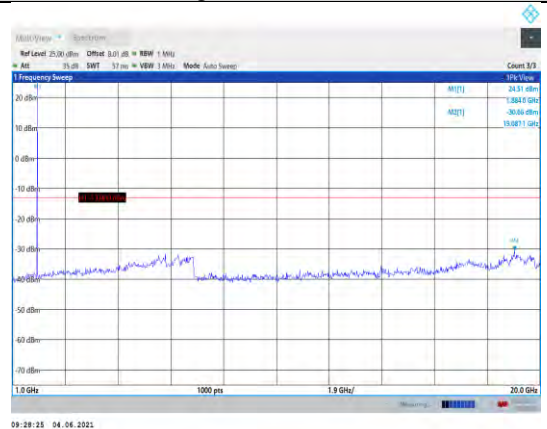
Band25-3MHz-QPSK-26365-1RB#0- Range2:1000~20000MHz
