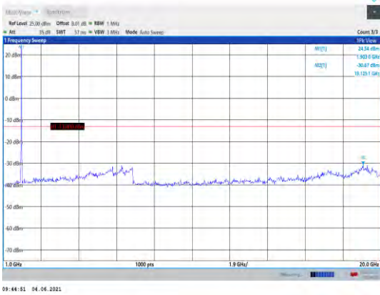
Band25-20MHz-QPSK-26590-1RB#0- Range2:1000~20000MHz
