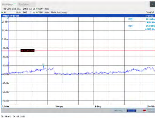
Band25-10MHz-QPSK-26090-1RB#0- Range2:1000~20000MHz
