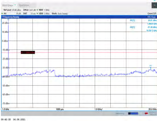
Band25-20MHz-QPSK-26140-1RB#0- Range2:1000~20000MHz
