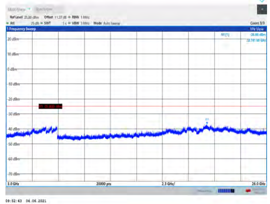
Band41-10MHz-QPSK-39700-1RB#0- Range3:3000~26000MHz
