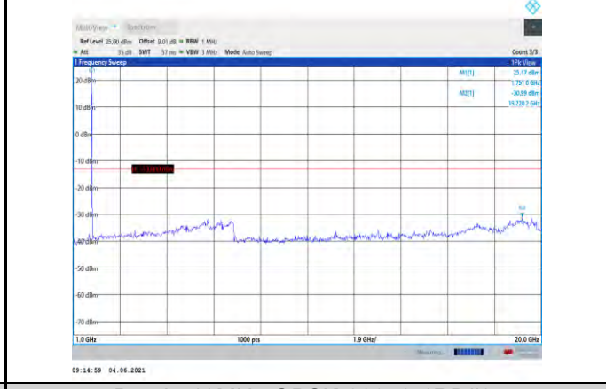
Band4-10MHz-QPSK-20350-1RB#0- Range2:1000~20000MHz
