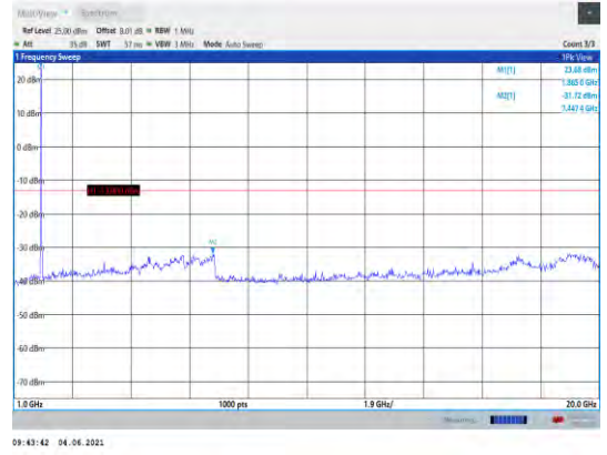
Band25-20MHz-QPSK-26365-1RB#0- Range2:1000~20000MHz
