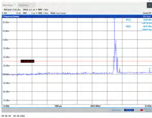
Band41-10MHz-QPSK-39700-1RB#0- Range2:1000~3000MHz
