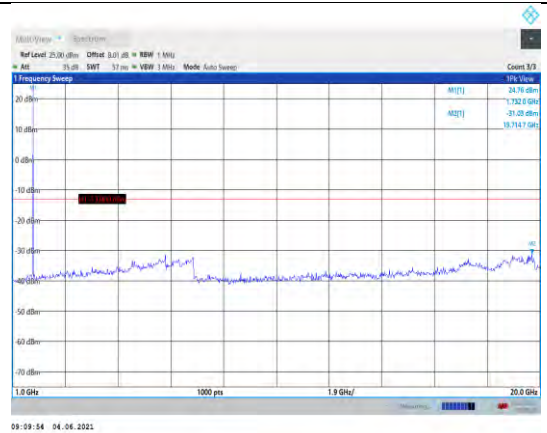
Band4-5MHz-QPSK-20175-1RB#0- Range2:1000~20000MHz
