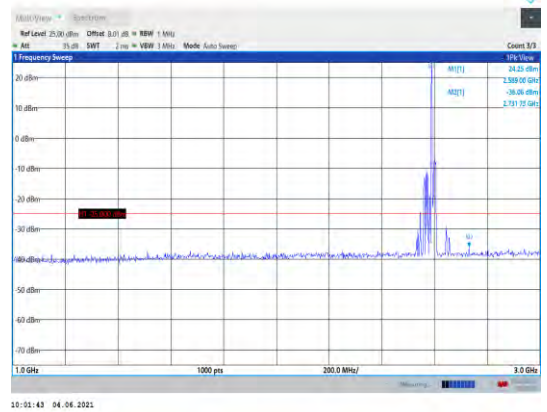
Band41-10MHz-QPSK-40620-1RB#0- Range2:1000~3000MHz
