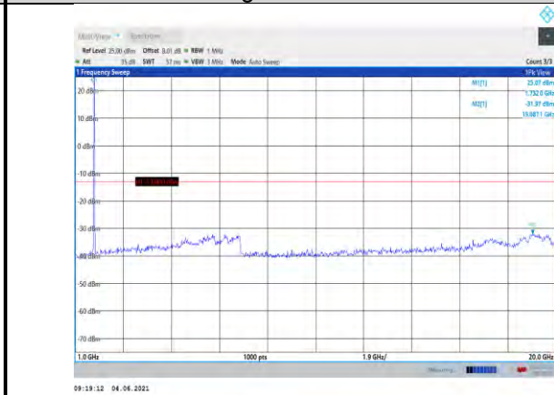
Band4-15MHz-QPSK-20325-1RB#0- Range2:1000~20000MHz
