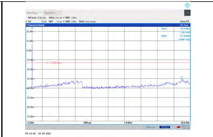
Band4-10MHz-QPSK-20175-1RB#0- Range2:1000~20000MHz
