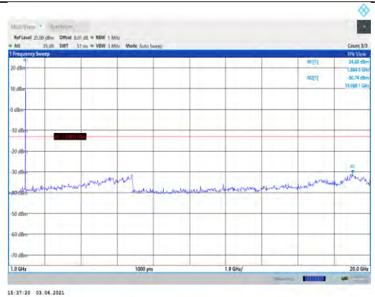
Band2-5MHz-QPSK-18900-1RB#0- Range2:1000~20000MHz
