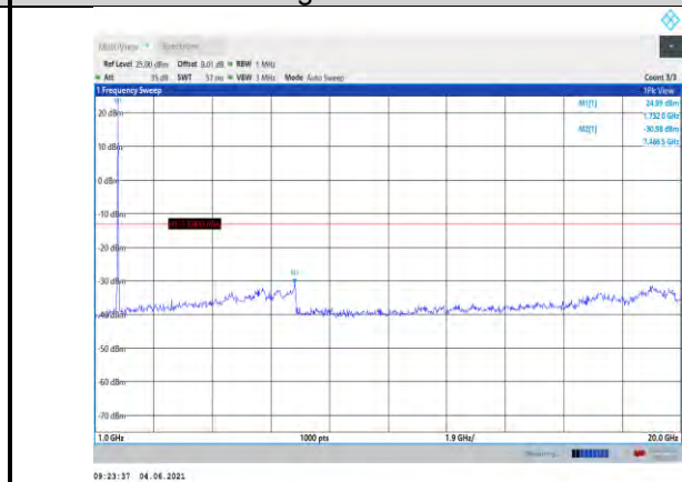
Band4-20MHz-QPSK-20300-1RB#0- Range2:1000~20000MHz
