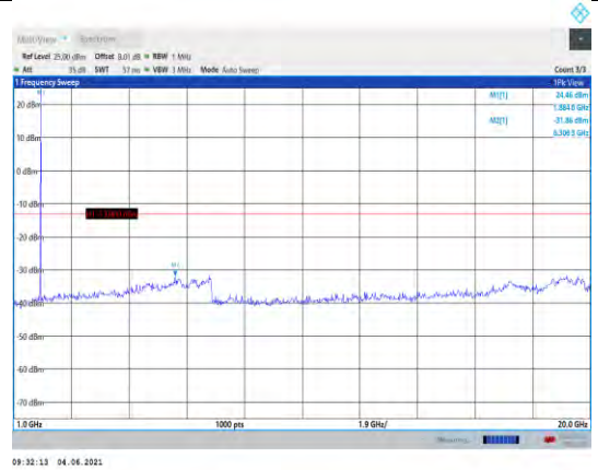
Band25-5MHz-QPSK-26365-1RB#0- Range2:1000~20000MHz
