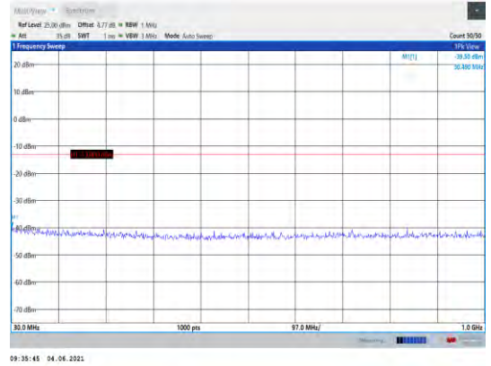
Band25-10MHz-QPSK-26365-1RB#0- Range1:30~1000MHz
