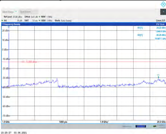
Band2-3MHz-QPSK-18615-1RB#0- Range2:1000~20000MHz
