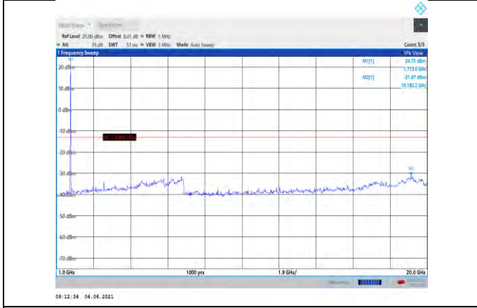
Band4-10MHz-QPSK-20000-1RB#0- Range2:1000~20000MHz
