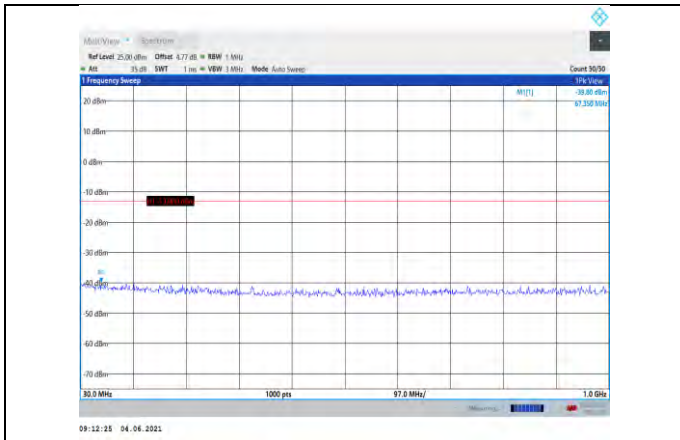
Band4-10MHz-QPSK-20000-1RB#0- Range1:30~1000MHz
