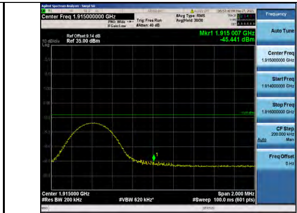
Band25-10MHz-QPSK-26640-1RB#0
