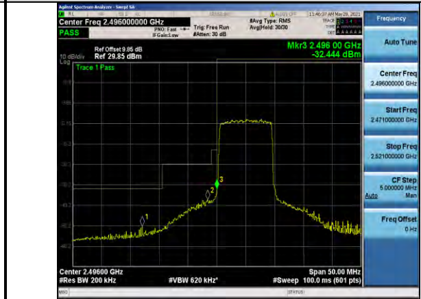
Band41-10MHz-QPSK-39700-50RB#0
