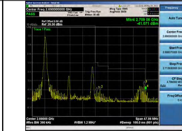
Band41-20MHz-QPSK-41490-1RB#0
