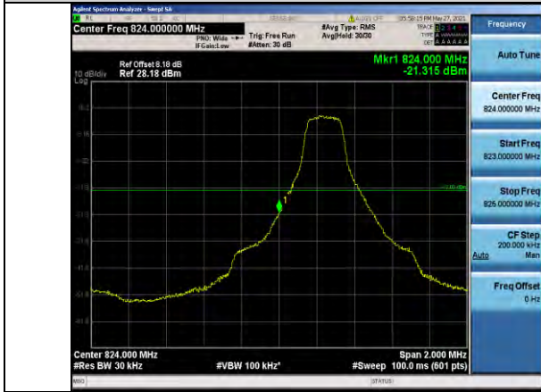
Band5-3MHz-QPSK-20415-1RB#0
