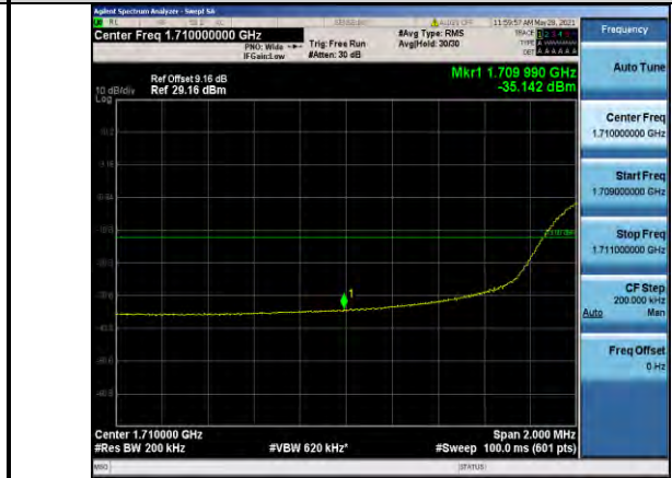
Band4-20MHz-QPSK-20050-100RB#0
