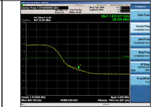
Band25-10MHz-QPSK-26640-50RB#0
