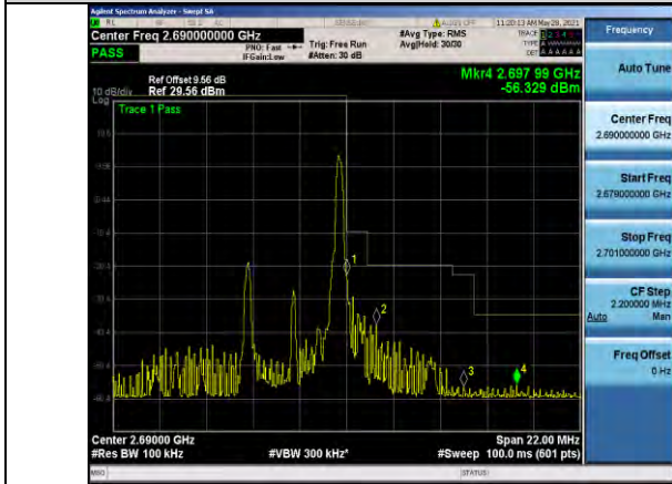
Band41-5MHz-16QAM-41565-1RB#24
