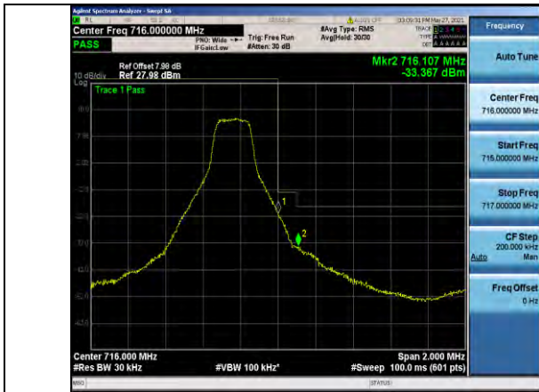
Band12-3MHz-QPSK-23165-1RB#14
