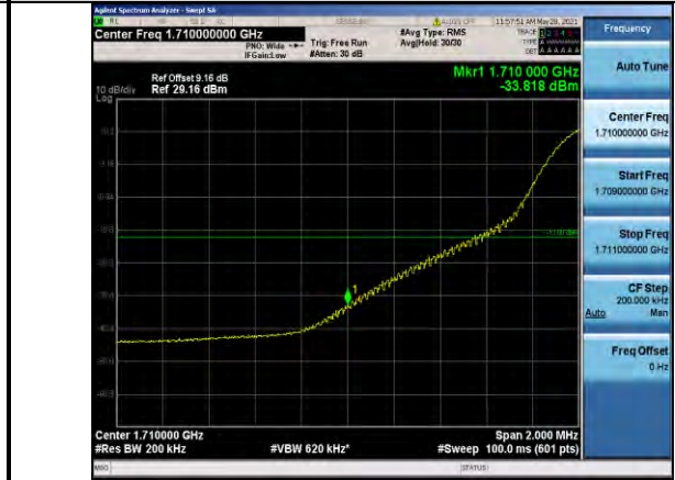
Band4-20MHz-QPSK-20050-1RB#0
