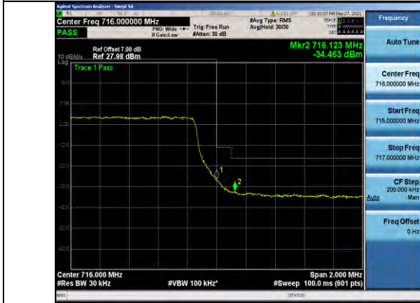
Band12-3MHz-QPSK-23165-15RB#0
