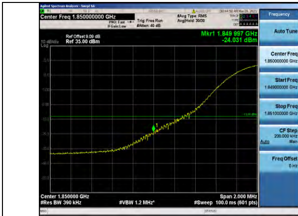
Band25-20MHz-QPSK-26140-1RB#0
