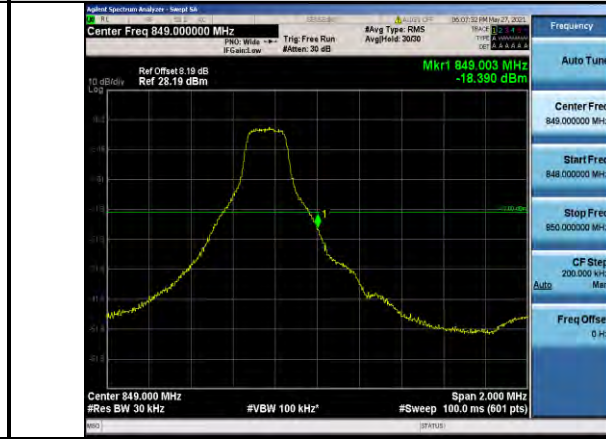
Band5-3MHz-QPSK-20635-1RB#14
