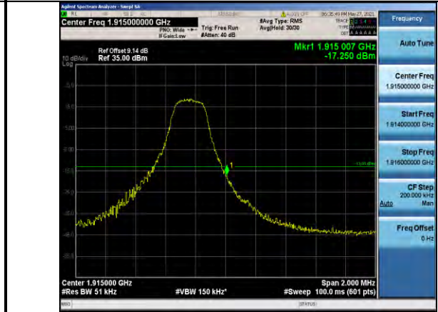
Band25-3MHz-QPSK-26675-1RB#14
