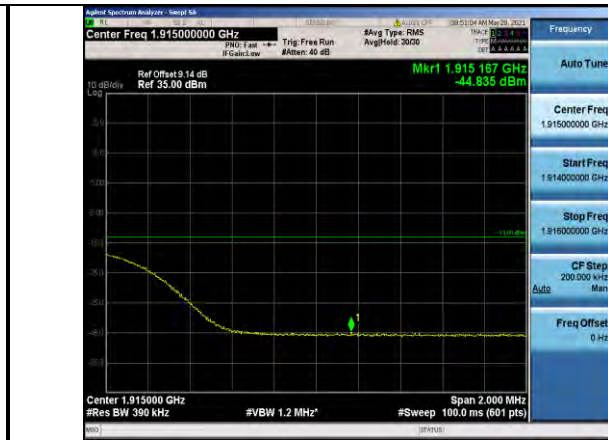
Band25-20MHz-16QAM-26590-1RB#0
