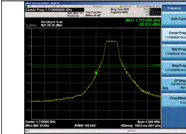
Band4-3MHz-QPSK-19965-1RB#0
