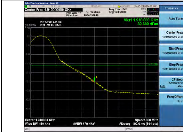
Band2-15MHz-16QAM-19125-1RB#74
