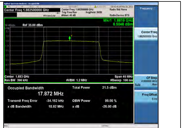
Band25-20MHz-QPSK-26365-100RB#0-17.872
