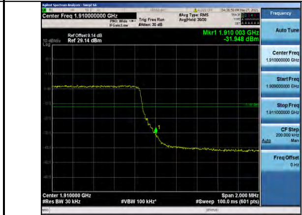
Band2-3MHz-QPSK-19185-15RB#0
