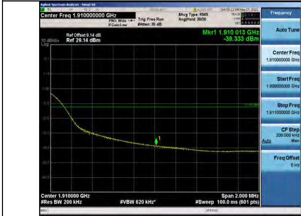
Band2-20MHz-QPSK-19100-100RB#0
