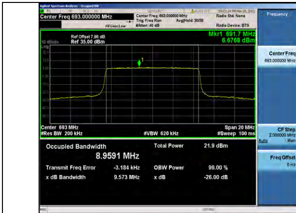
Band71-10MHz-QPSK-133422-50RB#0-8.9591
