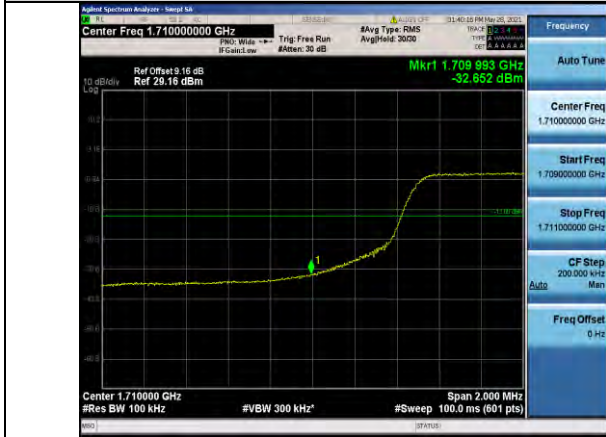
Band4-10MHz-QPSK-20000-50RB#0
