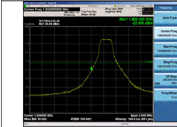
Band2-3MHz-QPSK-18615-1RB#0
