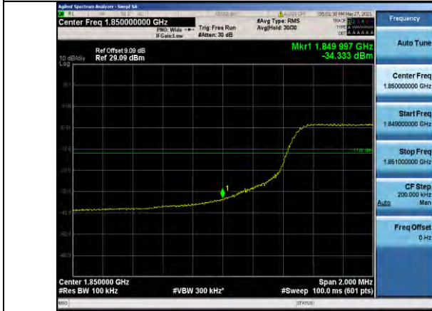
Band2-10MHz-QPSK-18650-50RB#0
