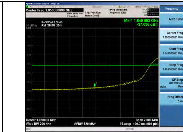
Band2-20MHz-16QAM-18700-100RB#0
