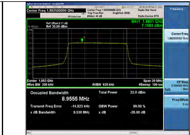
Band25-10MHz-QPSK-26365-50RB#0-8.9555
