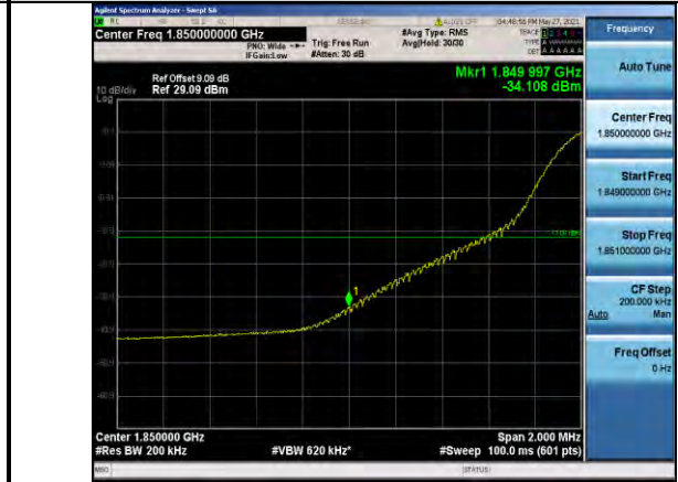
Band2-20MHz-QPSK-18700-1RB#0
