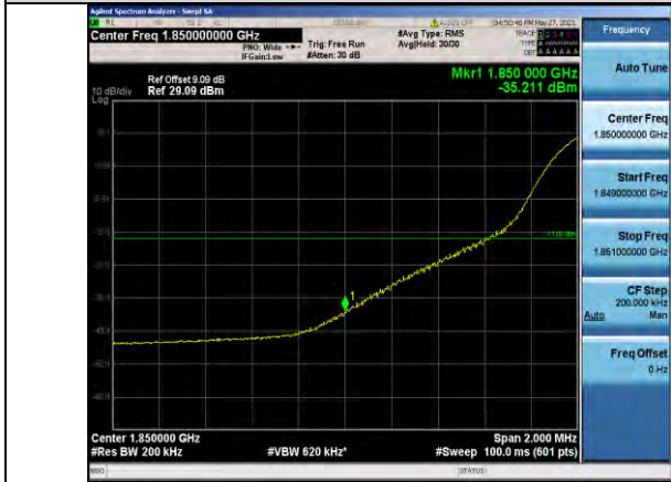
Band2-20MHz-16QAM-18700-1RB#0
