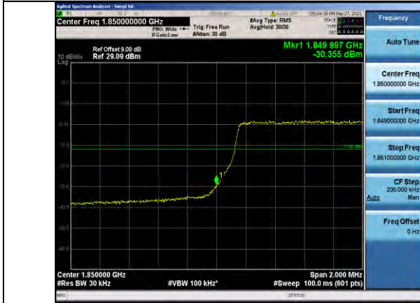
Band2-3MHz-16QAM-18615-15RB#0
