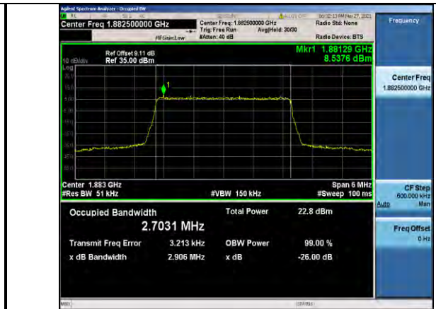
Band25-3MHz-QPSK-26365-15RB#0-2.7031
