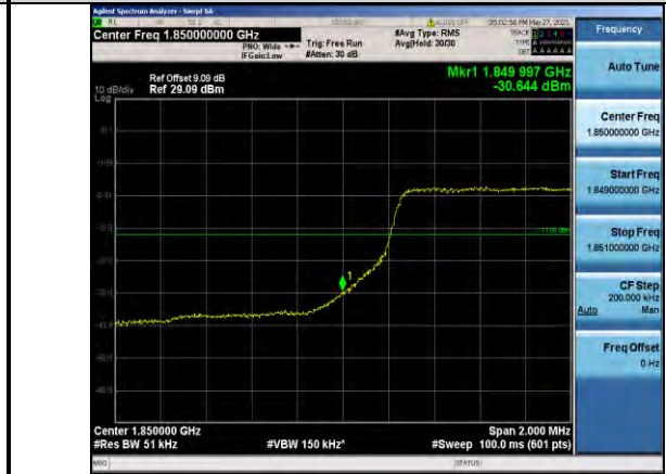
Band2-5MHz-QPSK-18625-25RB#0
