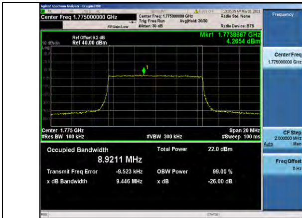
Band66-10MHz-QPSK-132622-50RB#0-8.9211
