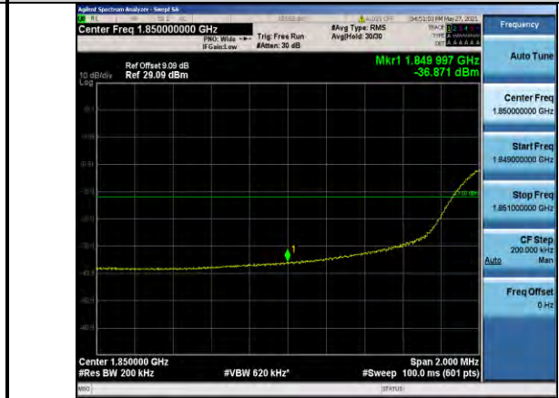
Band2-20MHz-QPSK-18700-100RB#0
