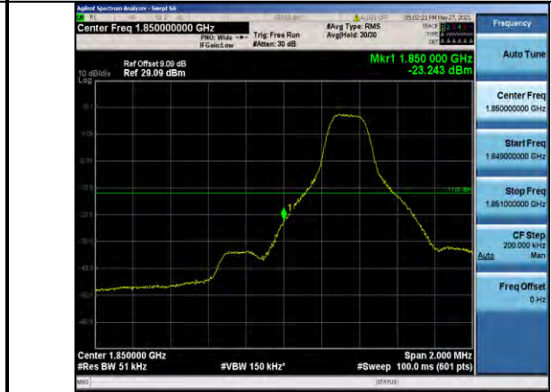
Band2-5MHz-QPSK-18625-1RB#0
