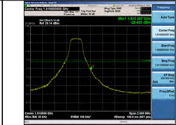
Band2-3MHz-QPSK-19185-1RB#14
