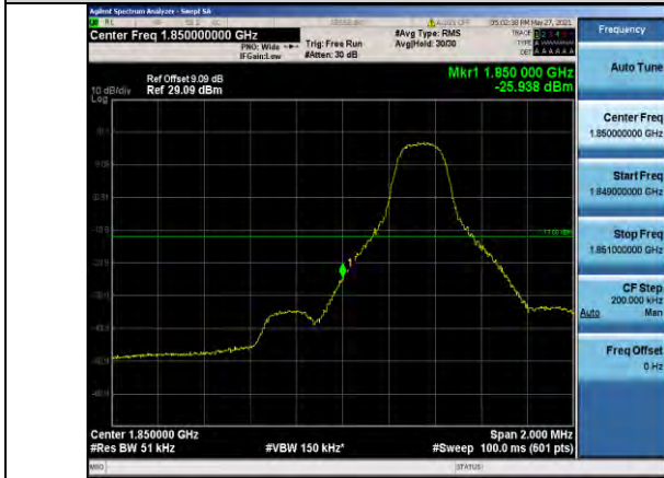
Band2-5MHz-16QAM-18625-1RB#0
