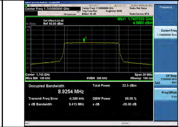
Band66-10MHz-QPSK-132322-50RB#0-8.9254
