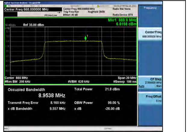
Band71-10MHz-QPSK-133172-50RB#0-8.9538
