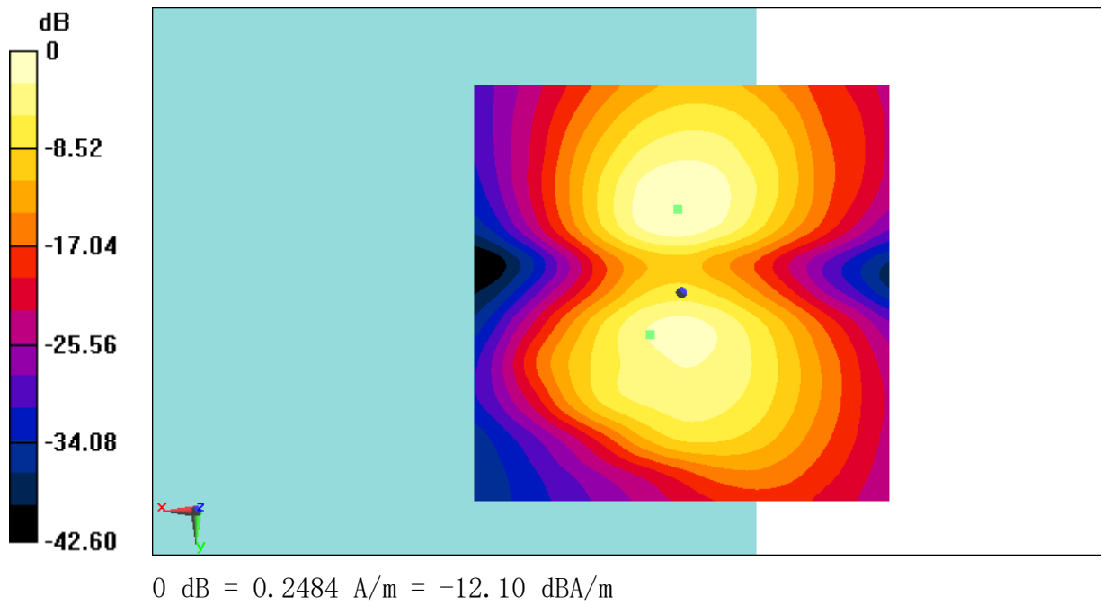
Fig B.9 T-Coil WCDMA 1700
