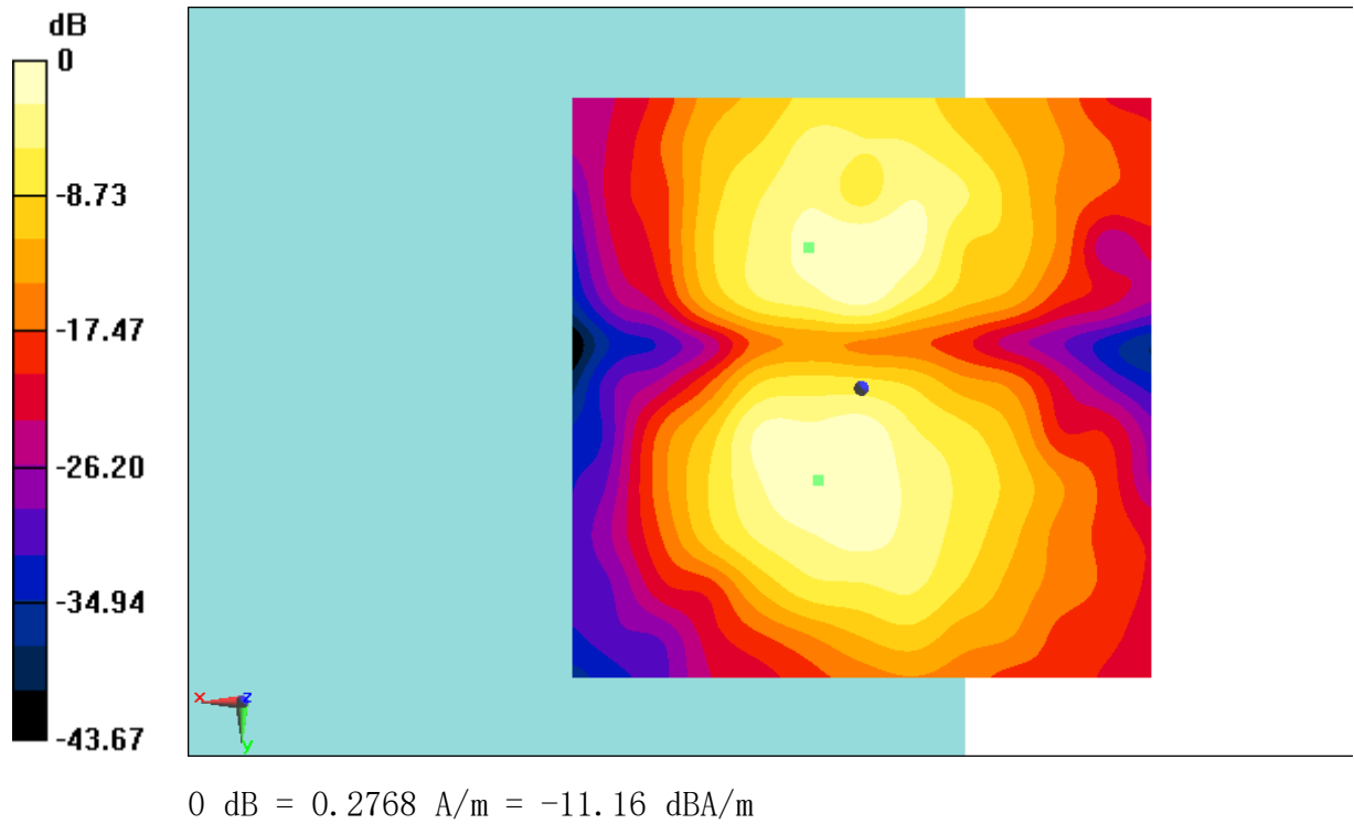
Fig B.41 T-Coil WiFi-2. 4G
