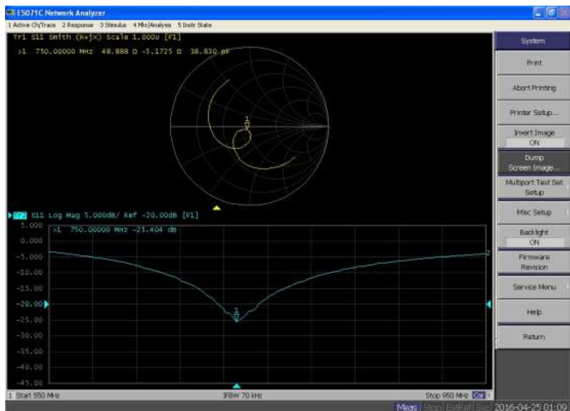
750MHz Body
