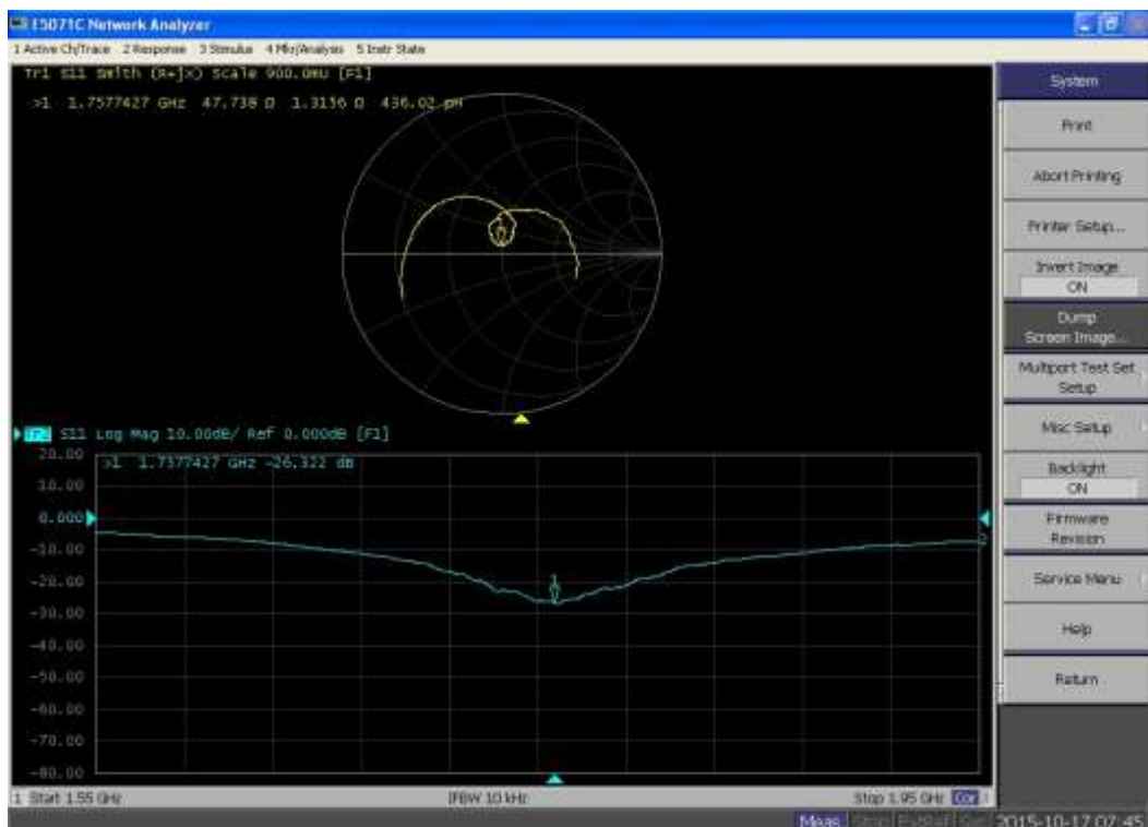
1750MHz Body
