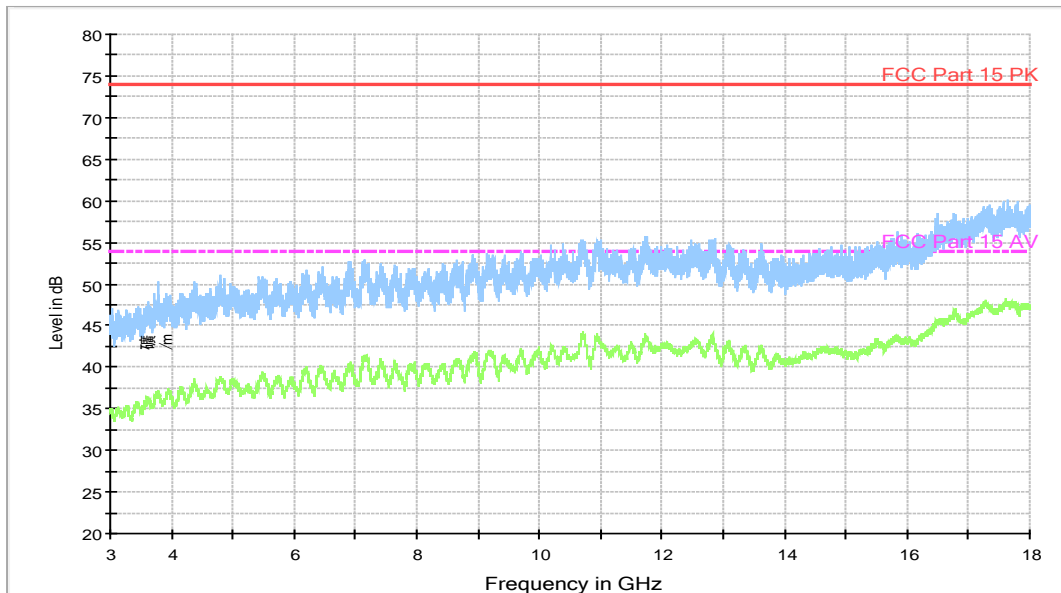
RE - 3GHz-18GHz
