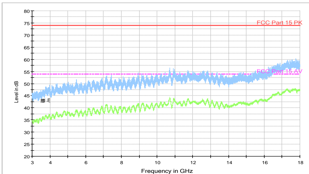
RE - 3GHz-18GHz
