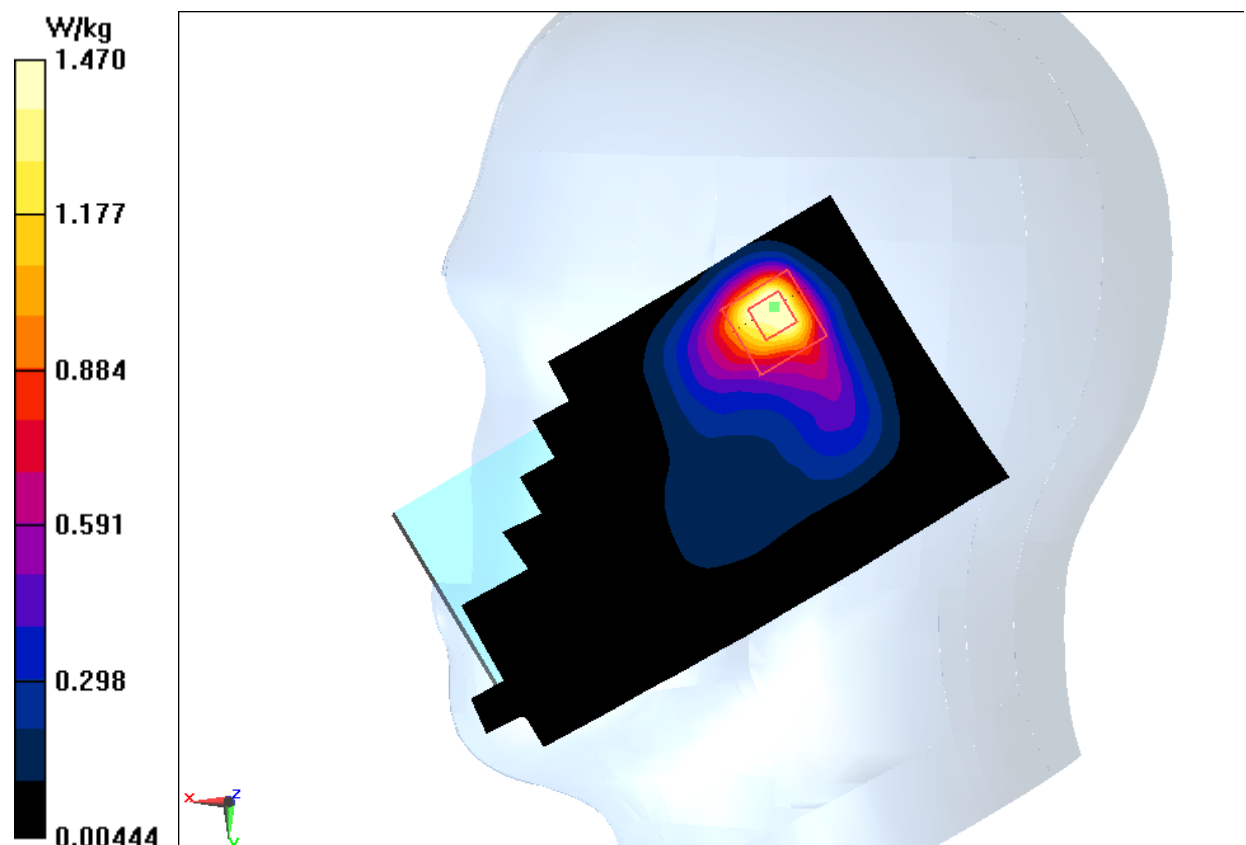
Fig.19 2450 MHz
