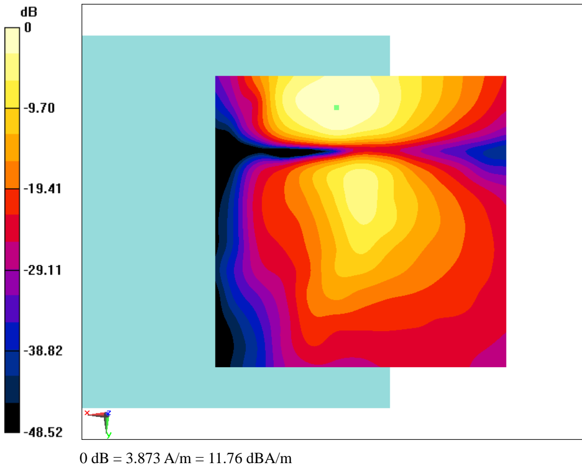
Fig B.6 T-Coil WCDMA 850
