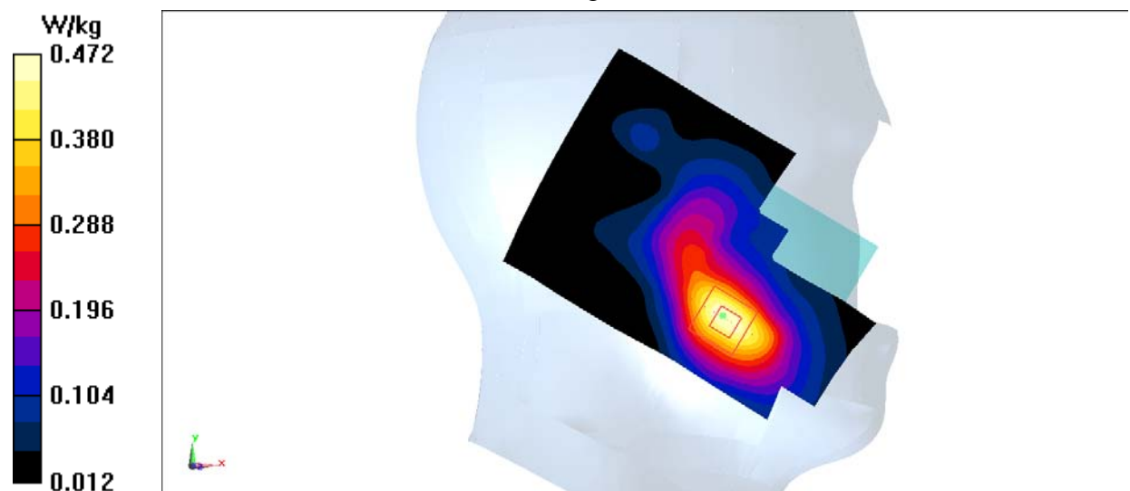
Fig.15 LTE Band4
