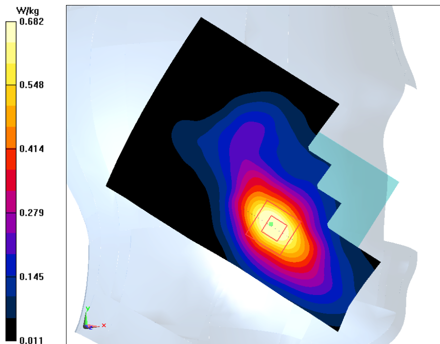
Fig.9 WCDMA1900
