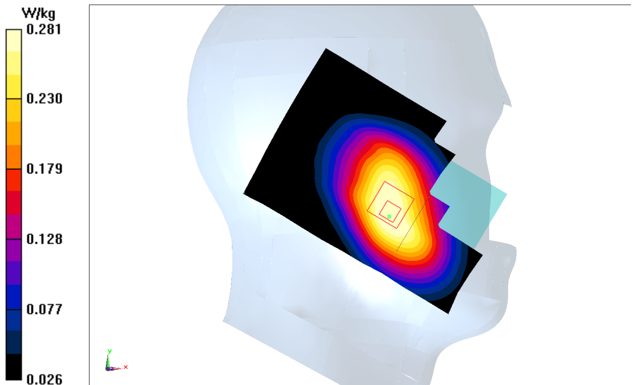
Fig.17 LTE Band5
