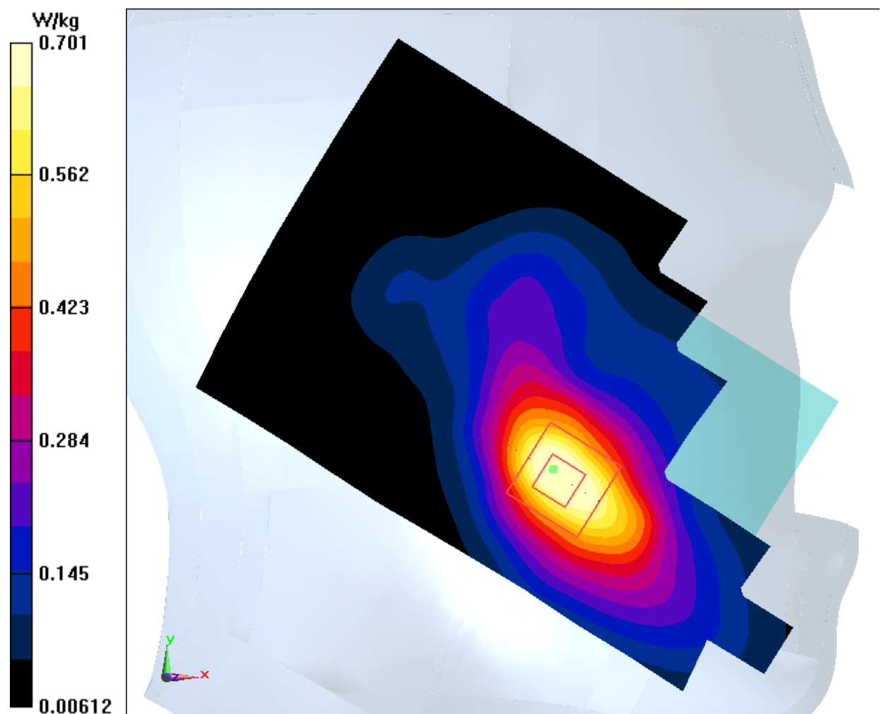
Fig.12 LTE Band2
