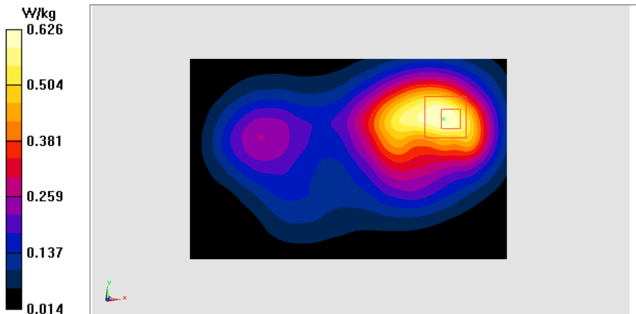
Fig.11 WCDMA1900
