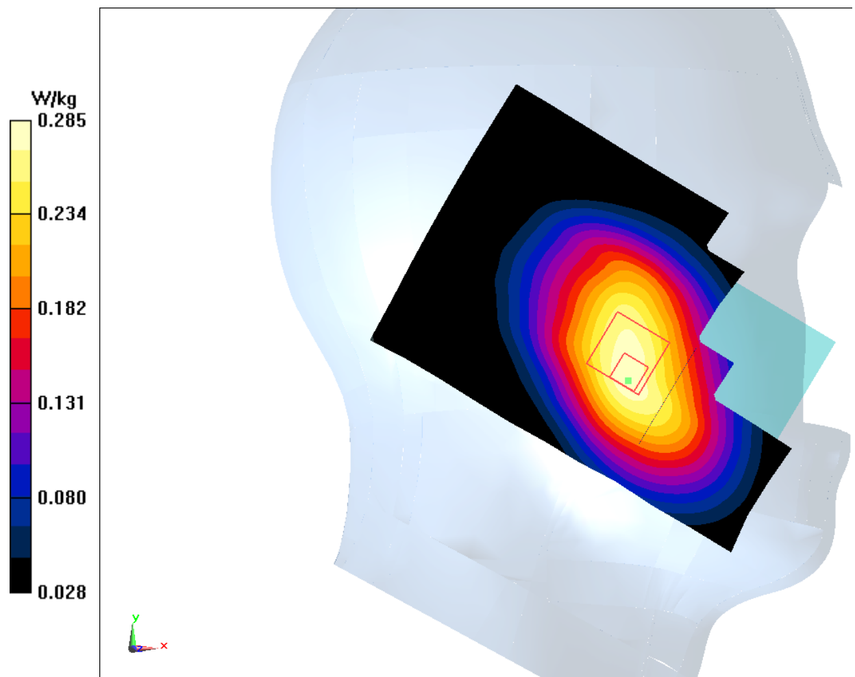
Fig.5 WCDMA 850
