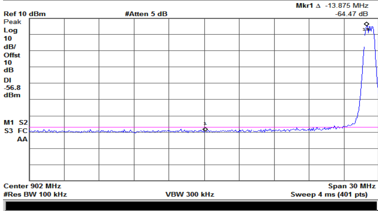
Plot 7 - Band Edge
