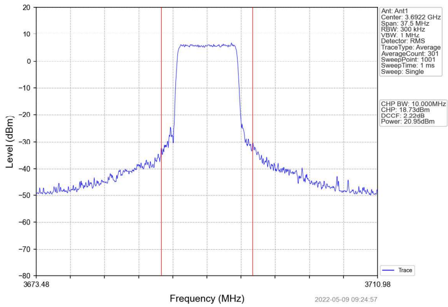
Band48_15MHz_QPSK_HCH_3692.5MHz_RB_36_39_NTNV
