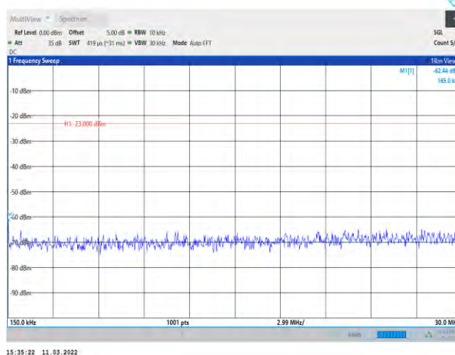
Band71-20MHz-QPSK-133222-1RB#0-Range2:0.15~30MHz
