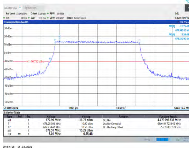
Band71-5MHz-QPSK-133297-25RB#0
