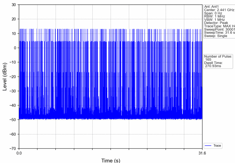
GFSK DH3_HOPP_Ant1_NTNV
