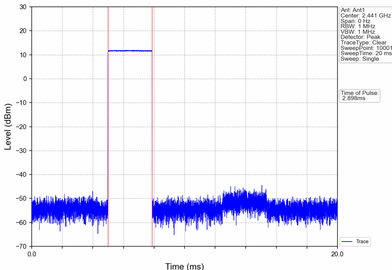
GFSK DH5_HOPP_Ant1_NTNV
