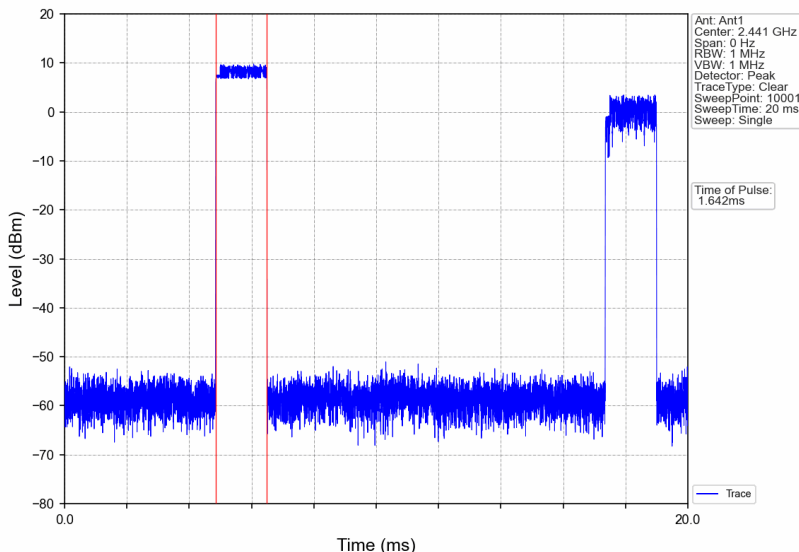
Pi/4DQPSK_2DH3_HOPP_Ant1_NTNV
