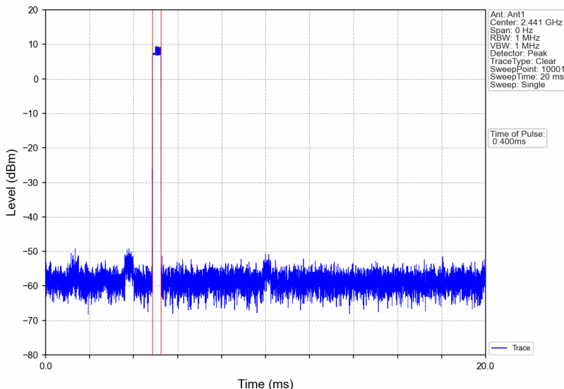
Pi/4DQPSK_2DH1_HOPP_Ant1_NTNV
