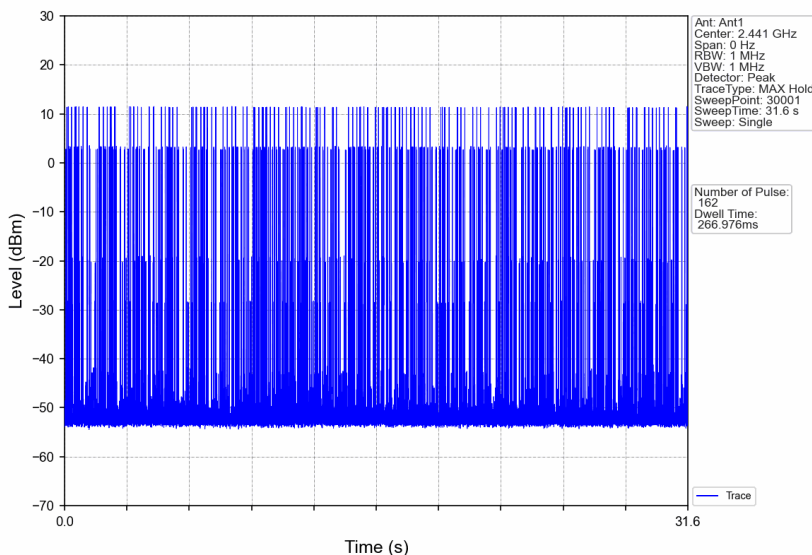
GFSK DH3_HOPP_Ant1_NTNV
