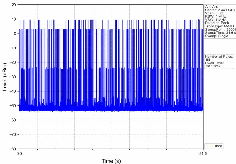
Pi/4DQPSK_2DH5_HOPP_Ant1_NTNV
