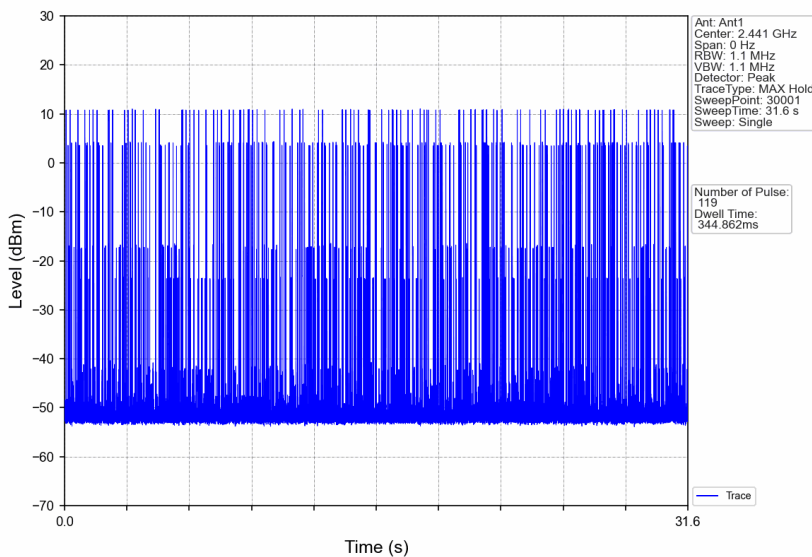
GFSK DH5_HOPP_Ant1_NTNV
