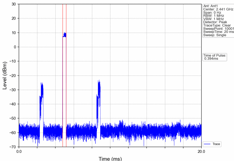
8DPSK 3DH1_HOPP_Ant1_NTNV
