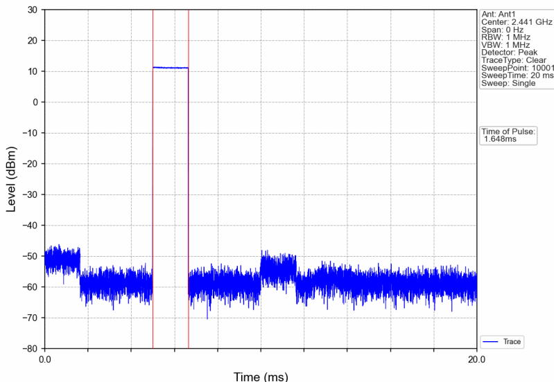
GFSK DH3_HOPP_Ant1_NTNV
