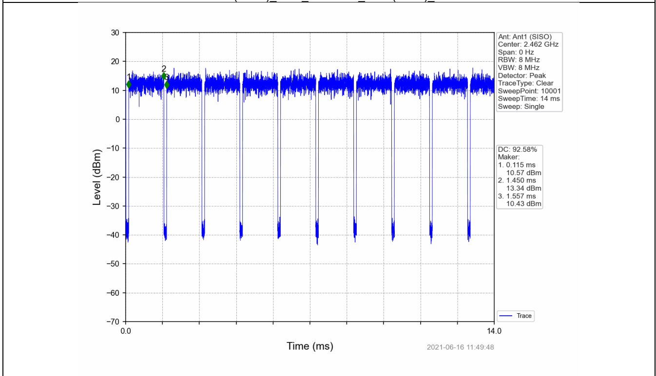
802.11n(HT20) HCH_2462MHz_Ant1 (SISO) NTVN
