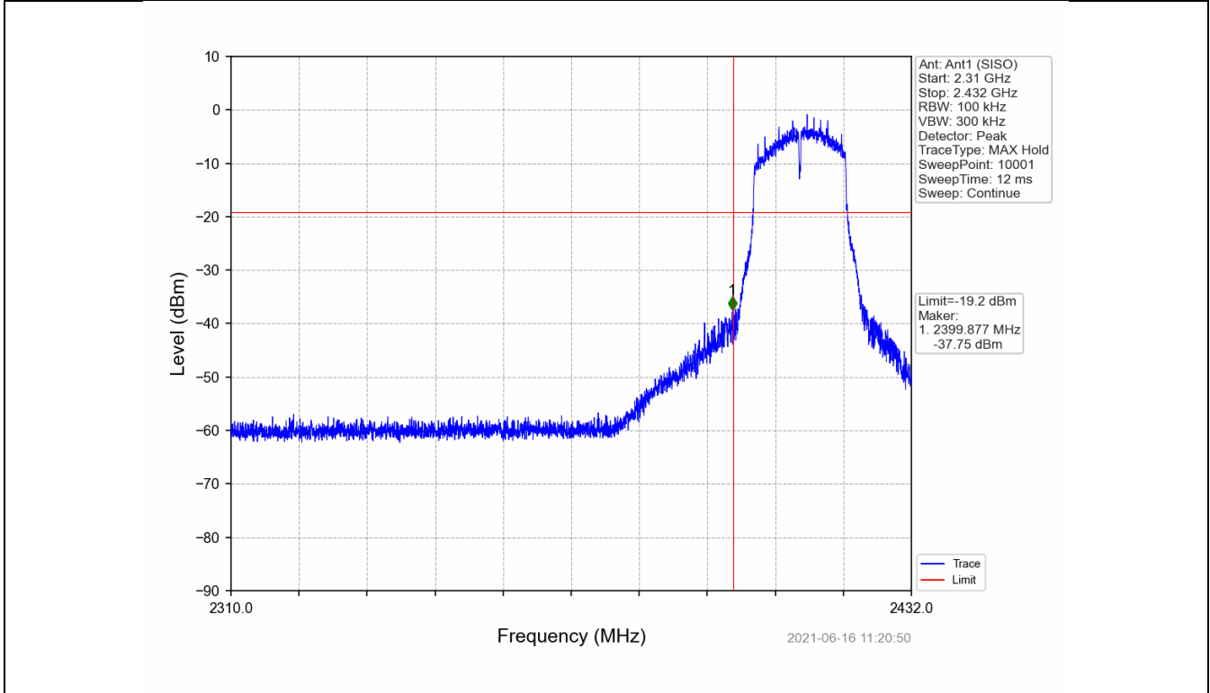
802.11g LCH 2412MHz Ant1 (SISO) NTN
