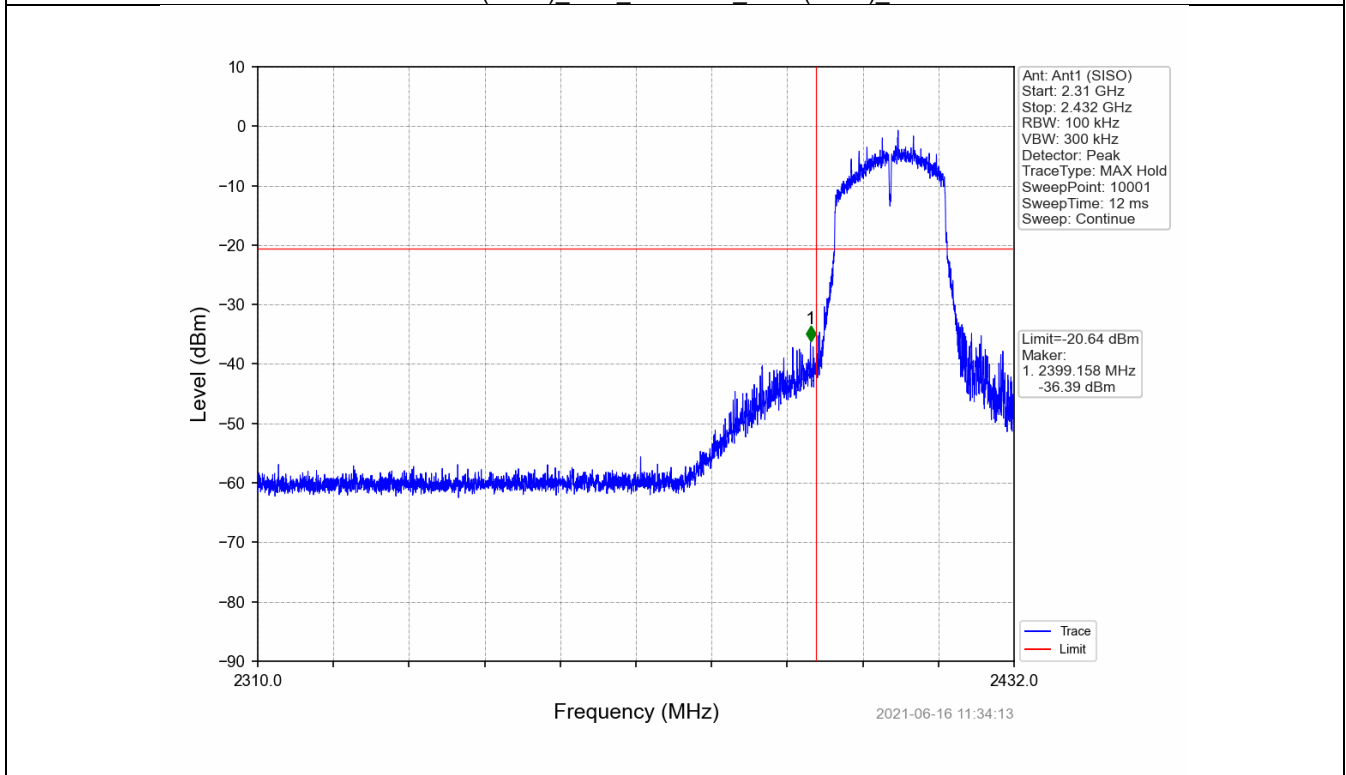
802.11n(HT20)_LCH_2412MHz_Ant1 (SISO)_NTNV
