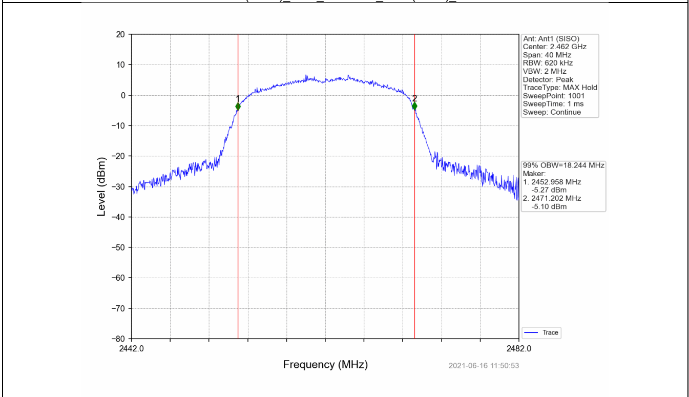
802.11n(HT20)_HCH_2462MHz_Ant1 (SISO)_NTNV
