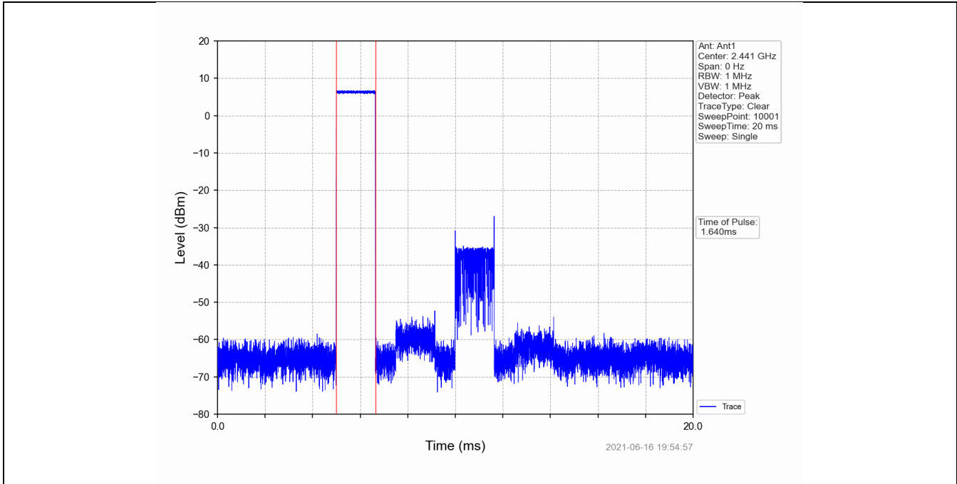
GFSK_DH3_HOPP_Ant1_NTNV
