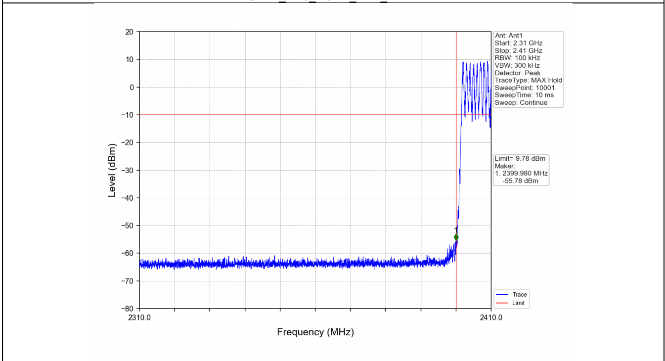
GFSK_DH5_HOPP_Ant1_NTNV
