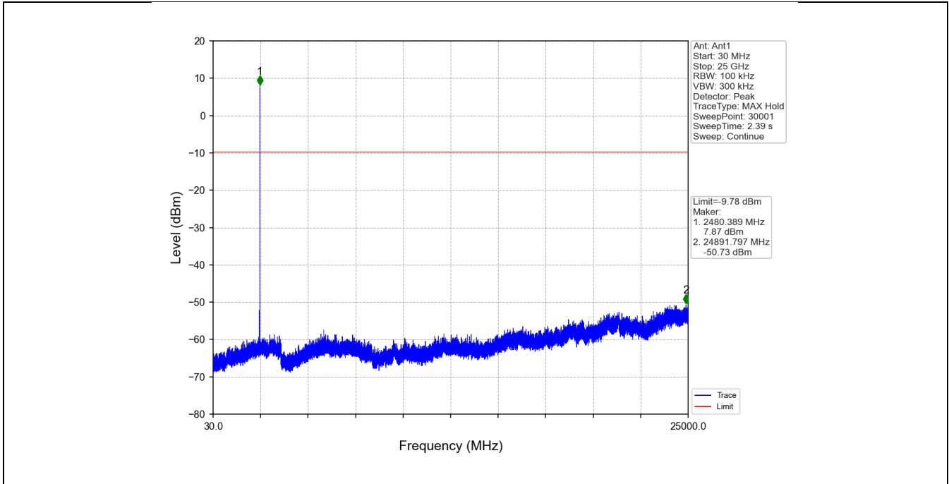
GFSK_DH5_HOPP_Ant1_NTNV
