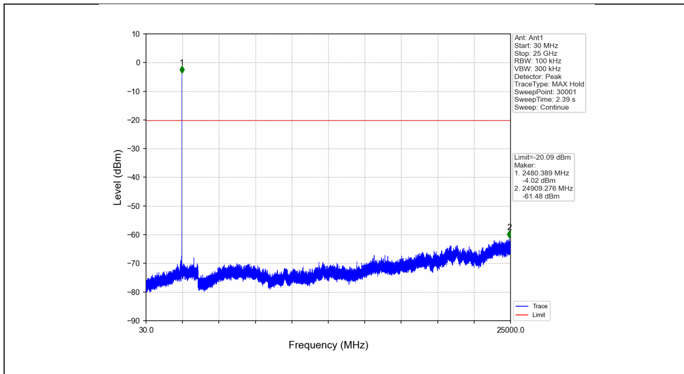
Pi/4DQPSK_2DH5_HOPP_Ant1_NTNV
