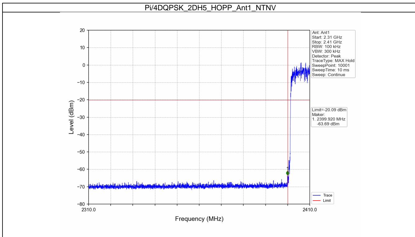
Pi/4DQPSK_2DH5_HOPP_Ant1_NTNV
