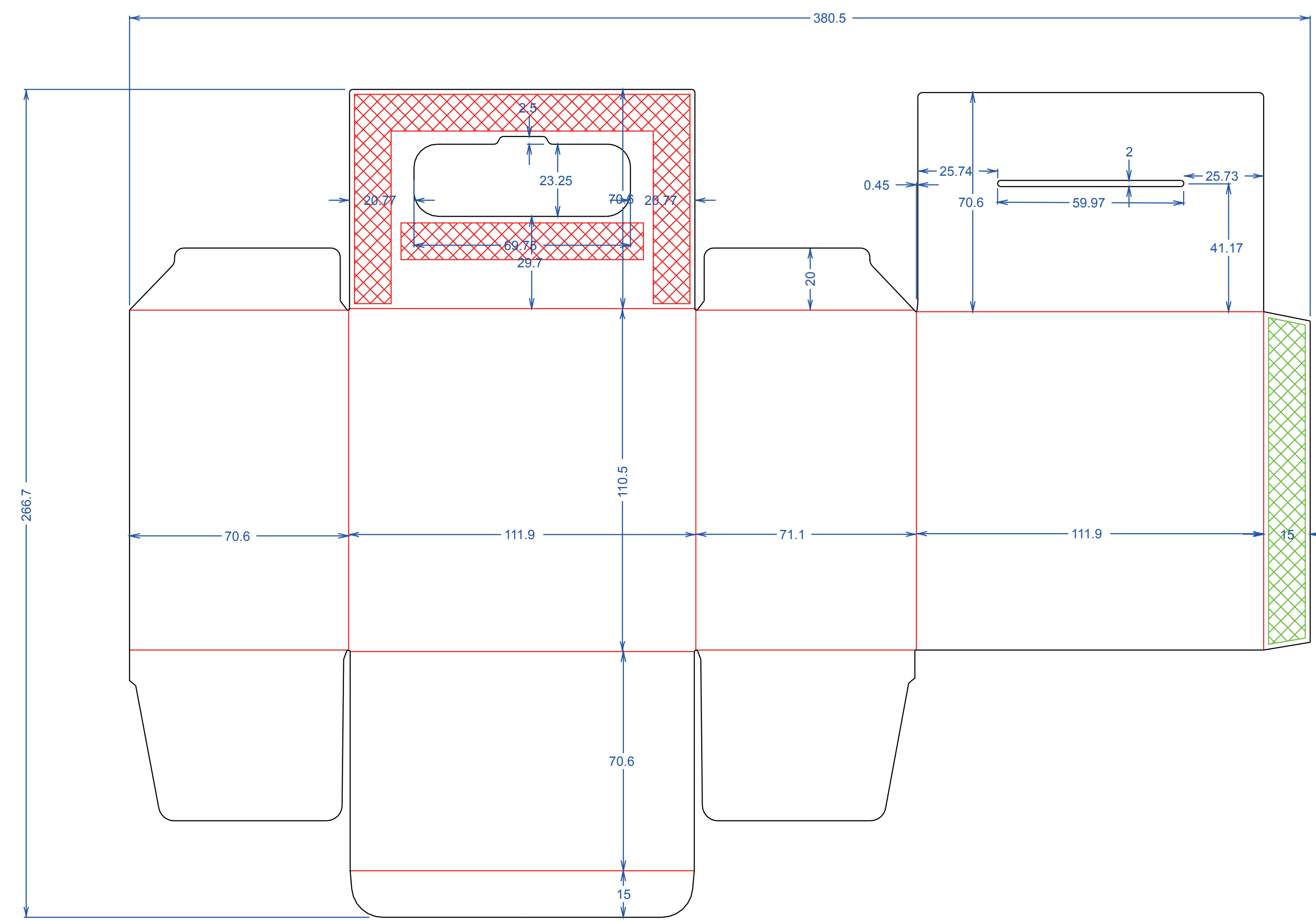
部件名称: GT通用封套 材质: 300g太阳白卡纸+PLA降解哑膜 工艺: 印刷+PLA降解哑膜+局部亮UV+3D立体击凸
