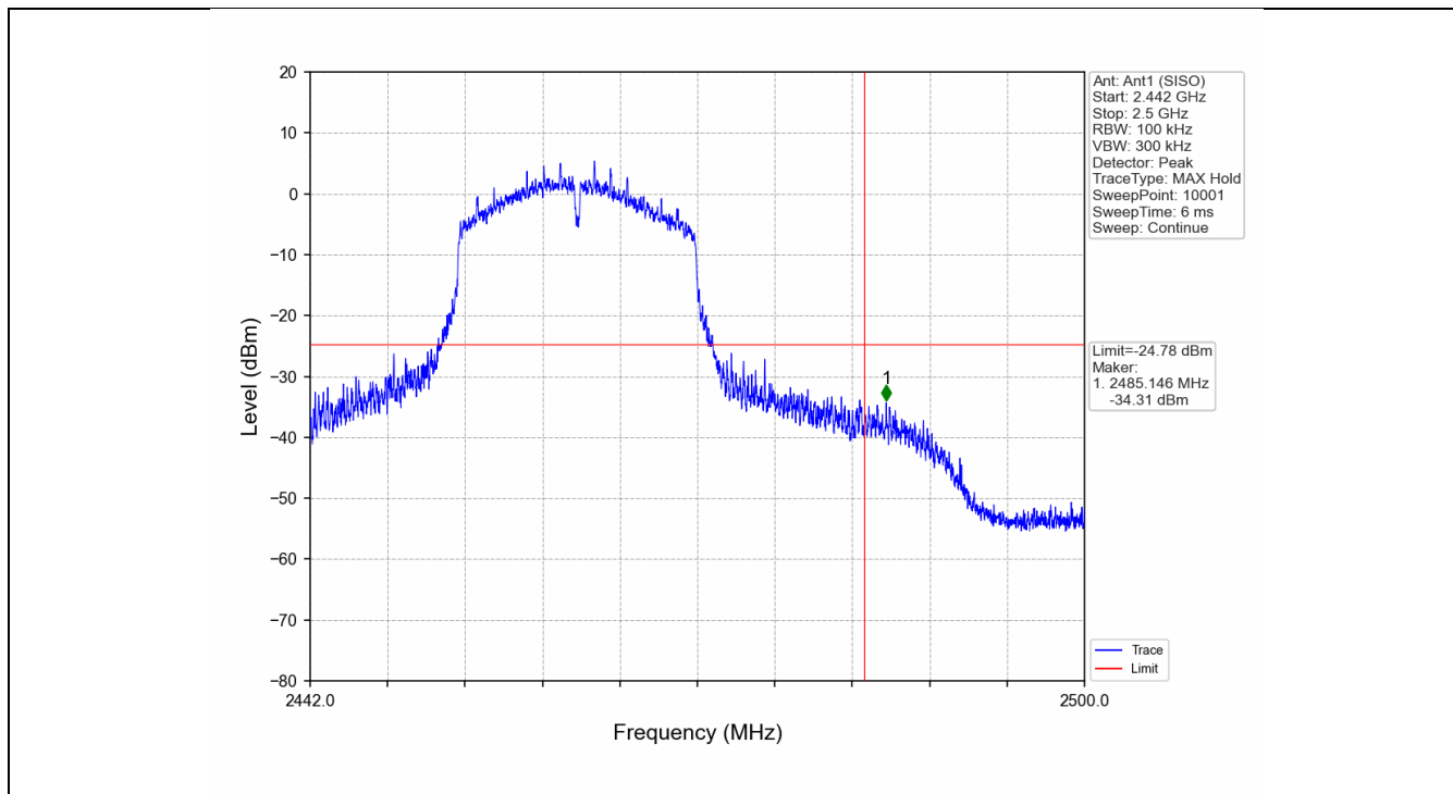
802.11n(HT20)_HCH_2462MHz_Ant1 (SISO)_NTNV
