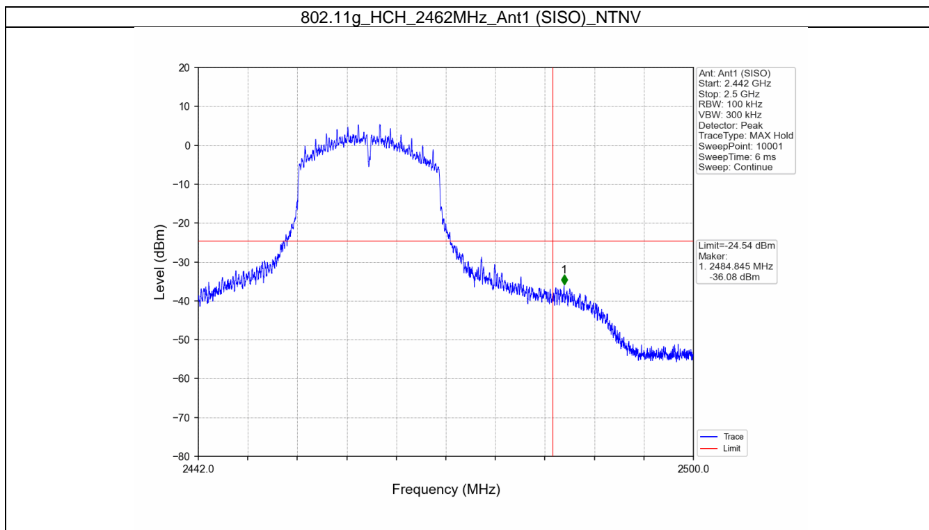
802.11g_HCH_2462MHz_Ant1 (SISO)_NTNV
