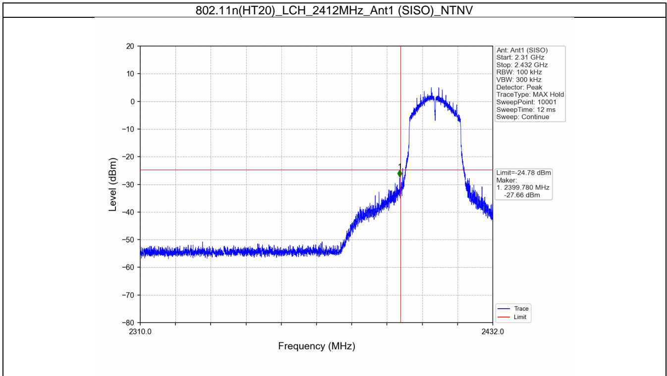
802.11n(HT20)_LCH_2412MHz_Ant1 (SISO)_NTNV
