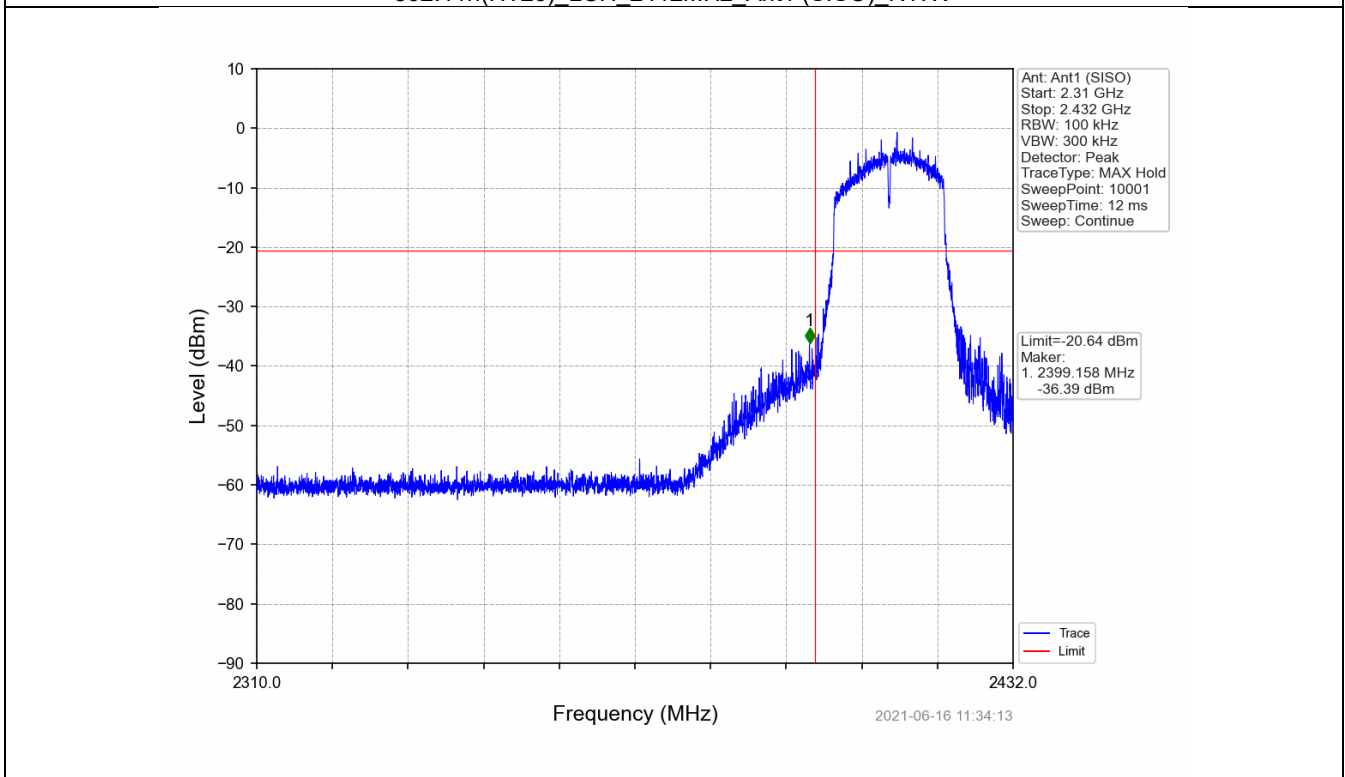
802.11n(HT20)_LCH_2412MHz_Ant1 (SISO)_NTNV
