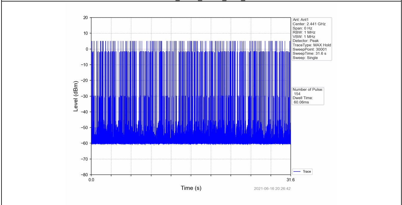
Pi/4DQPSK_2DH3_HOPP_Ant1_NTNV
