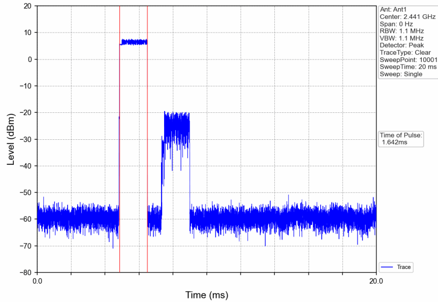
Pi/4DQPSK_2DH3_HOPP_Ant1_NTNV
