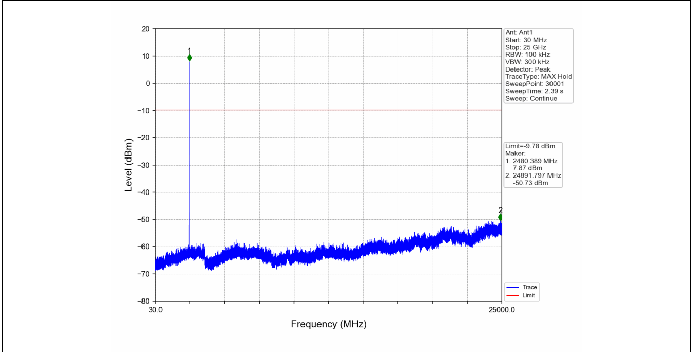
GFSK_DH5_HOPP_Ant1_NTNV
