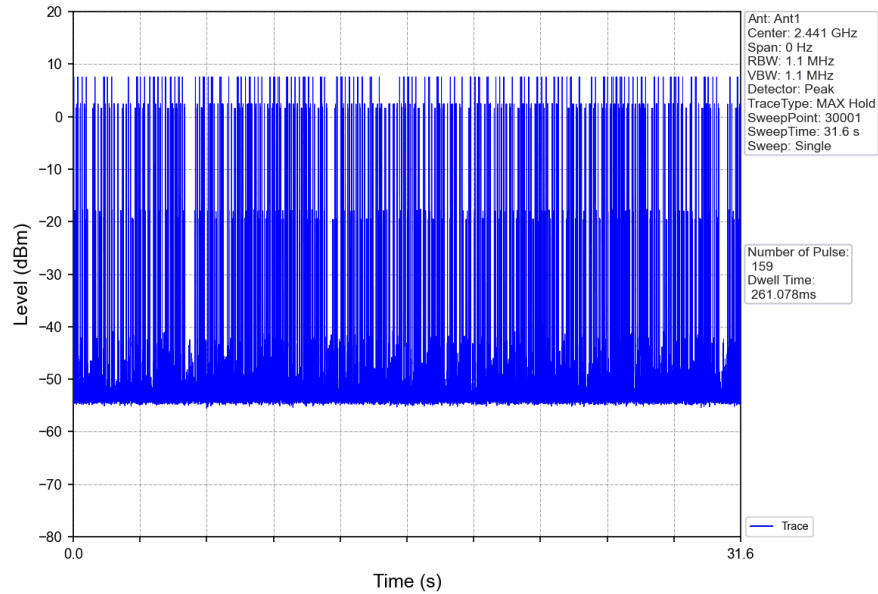
Pi/4DQPSK_2DH3_HOPP_Ant1_NTNV
