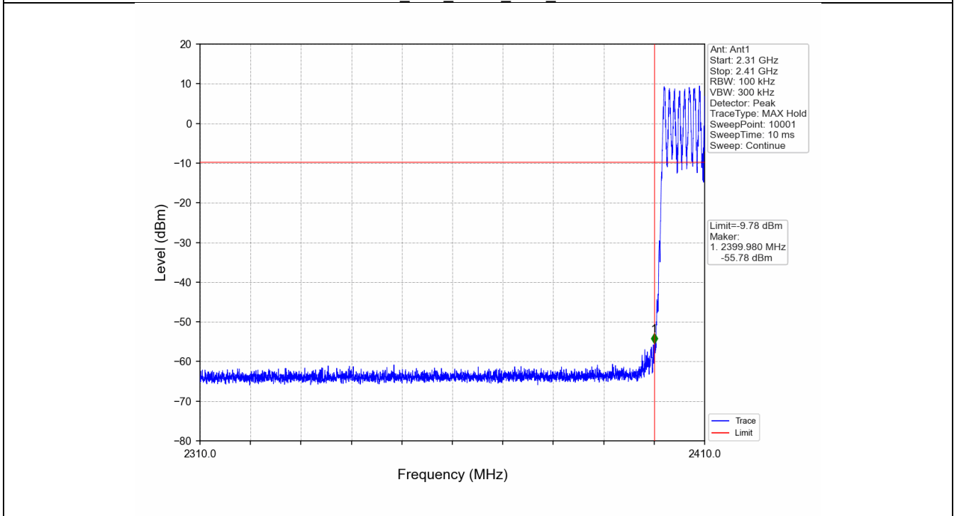
GFSK_DH5_HOPP_Ant1_NTNV
