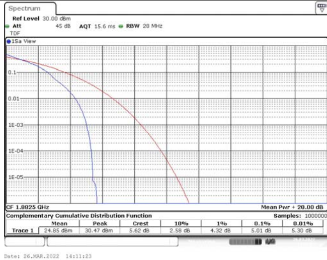
Band25-20MHz-QPSK-26365-1RB#0
