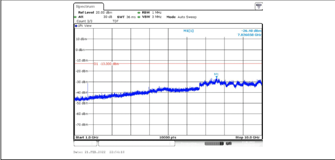
Band26-1.4MHz-QPSK-26697-1RB#0-Range2:1000~10000MHz
