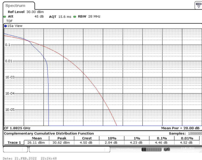
Band25-10MHz-16QAM-26365-1RB#0
