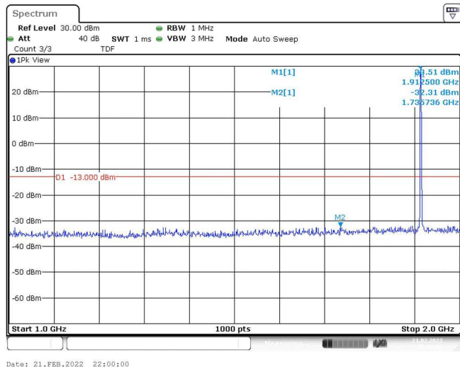
Band25-3MHz-QPSK-26675-1RB#0-Range2:1000~2000MHz
