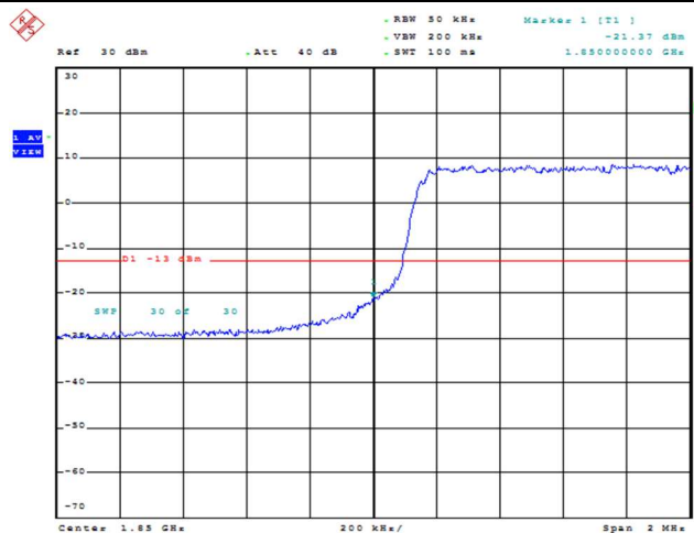
Band2-3MHz-QPSK-18615-1RB#14
