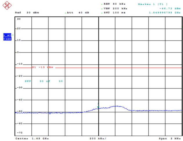
Band2-3MHz-QPSK-18615-1RB#0
