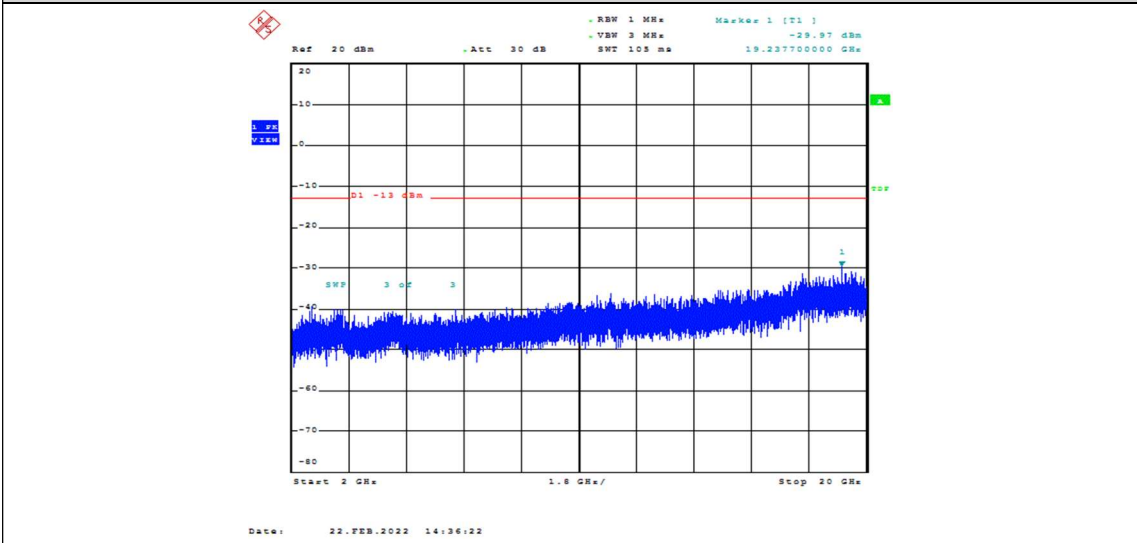
Band2-3MHz-QPSK-18615-1RB#0-Range3:2000~20000MHz
