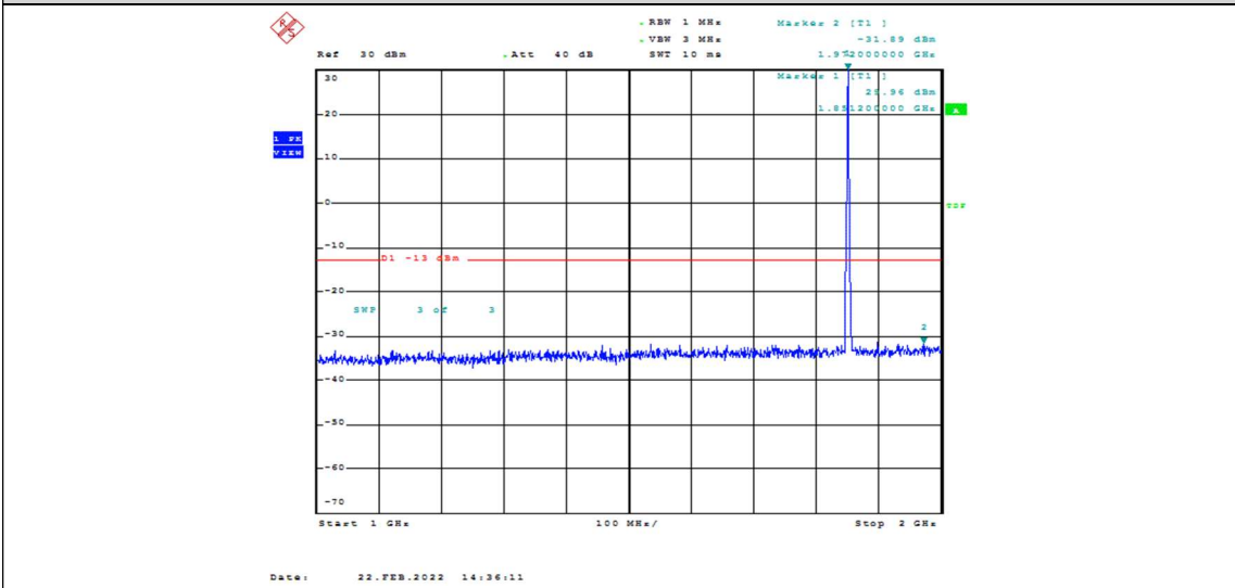
Band2-3MHz-QPSK-18615-1RB#0-Range2:1000~2000MHz
