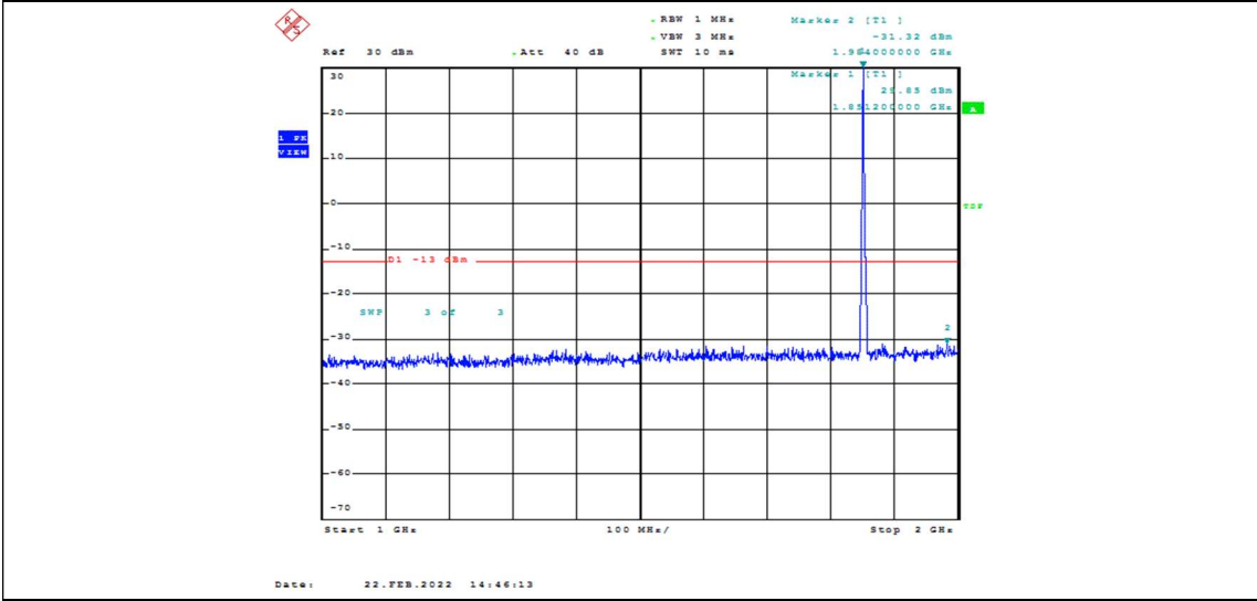
Band2-5MHz-QPSK-18625-1RB#0-Range2:1000~2000MHz
