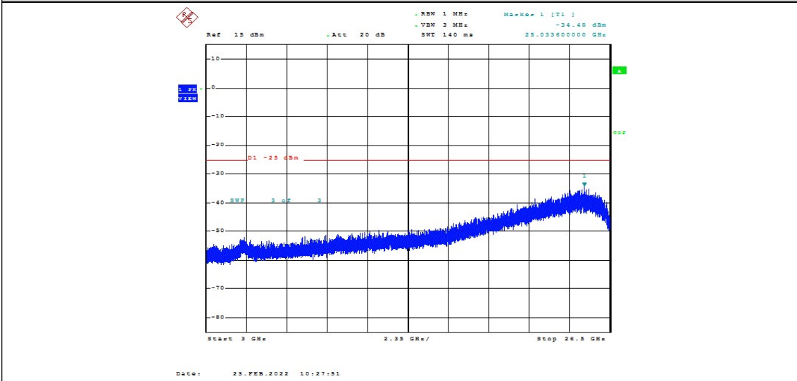
Band41-5MHz-QPSK-39675-1RB#0-Range1:3000~26500MHz
