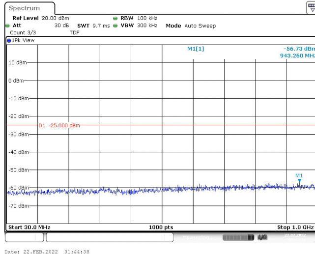
Band41-10MHz-QPSK-39700-1RB#0-Range1:30~1000MHz
