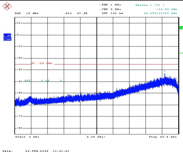
Band41-10MHz-QPSK-39700-1RB#0-Range1:3000~26500MHz
