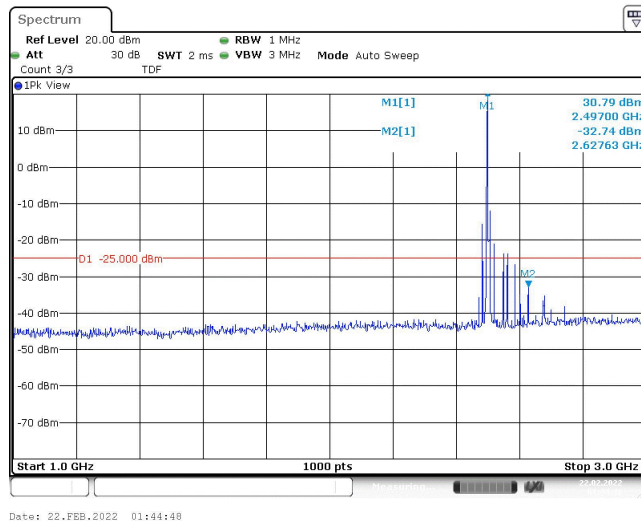
Band41-10MHz-QPSK-39700-1RB#0-Range2:1000~3000MHz
