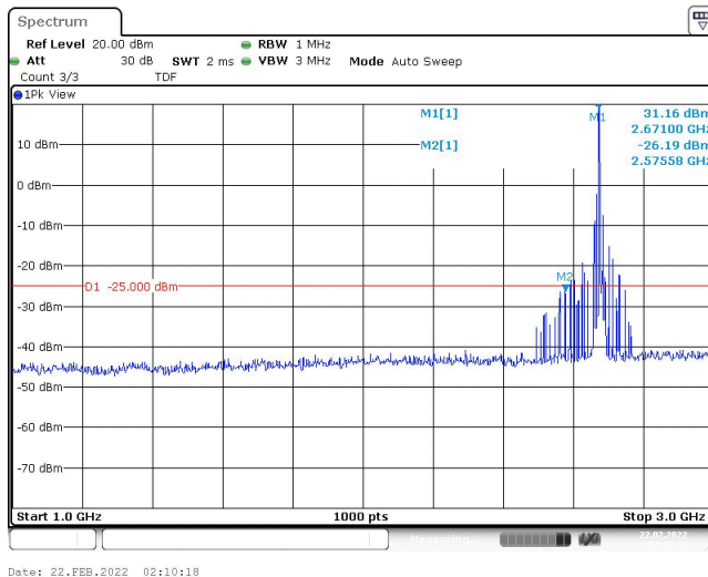
Band41-20MHz-QPSK-41490-1RB#0-Range2:1000~3000MHz
