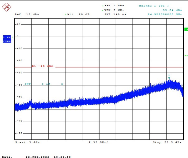
Band41-20MHz-QPSK-41490-1RB#0-Range1:3000~26500MHz
