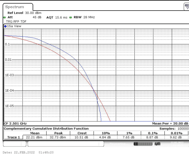
Band41-10MHz-QPSK-39700-50RB#0
