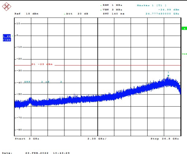
Band7-5MHz-QPSK-21425-1RB#0-Range1:3000~26500MHz
