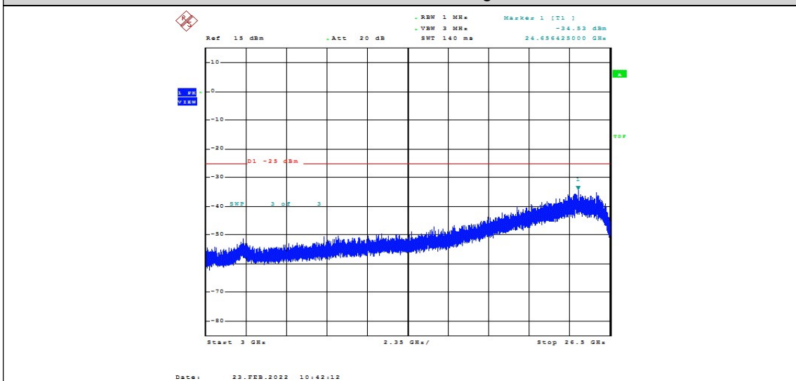
Band7-5MHz-QPSK-20775-1RB#0-Range1:3000~26500MHz
