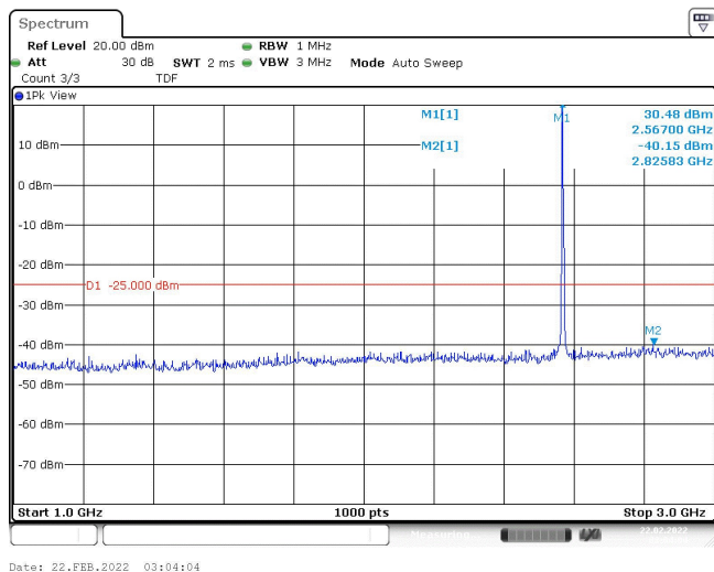
Band7-5MHz-QPSK-21425-1RB#0-Range2:1000~3000MHz
