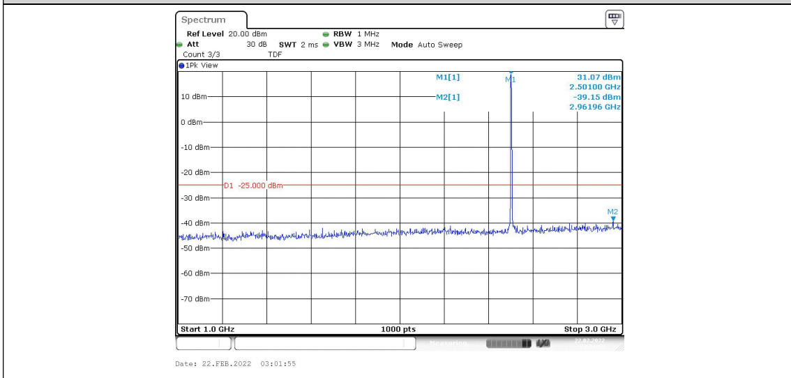
Band7-5MHz-QPSK-20775-1RB#0-Range2:1000~3000MHz
