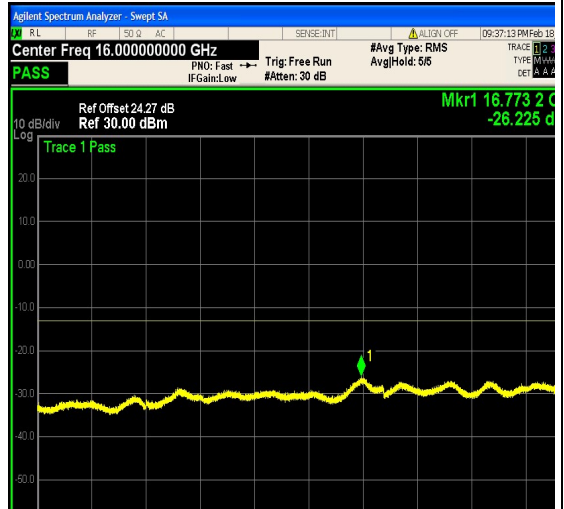
1-N25-PC3-15-20-M-16-CP-QPSK-Edge_1R B_Left-1@0-12000-20000-Ant1--26.22--13-PASS
