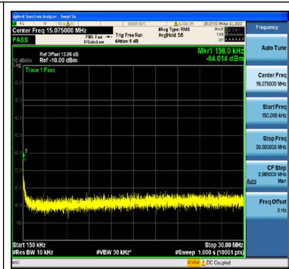
1-N2-PC3-15-5-L-4-DFT-QPSK-Edge_1RB_L eft-1@0-0.15-30-Ant1--64.01--33-PASS
