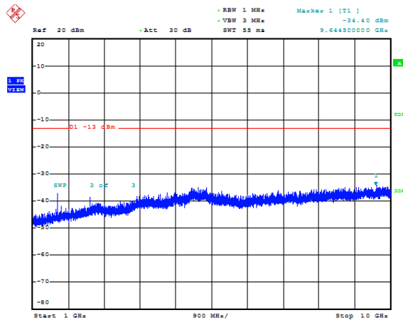
Band26-1.4MHz-QPSK-26697-1RB#0-Range2:1000~10000MHz
