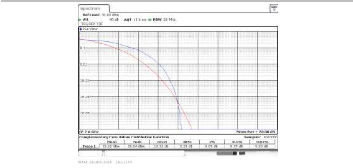
Band41_10MHz_QPSK_40690_1RB#0
