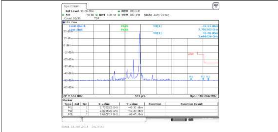
Band41_10MHz_QPSK_4190_50RB#0
