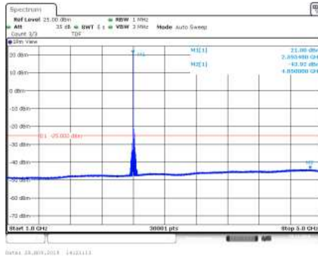
Band41_10MHz_QPSK_40690_1RB#0
