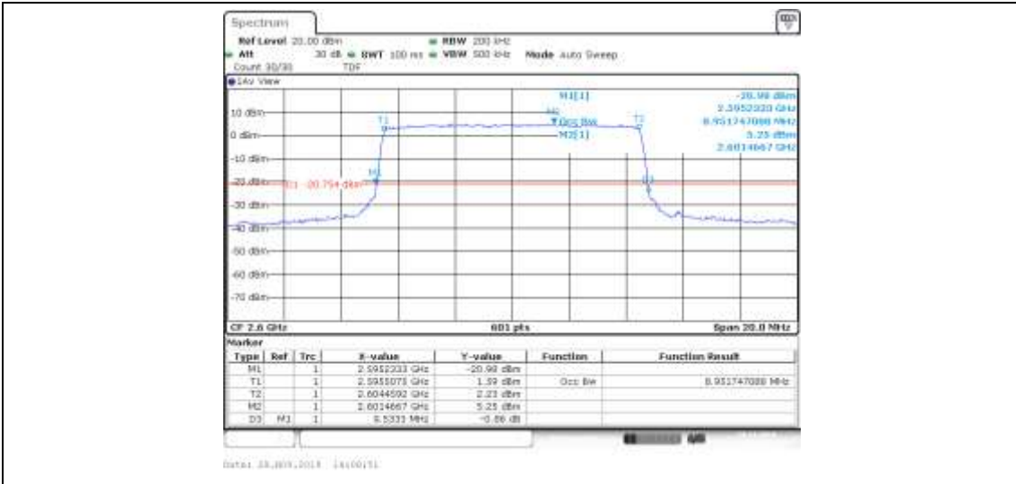
Band41_10MHz_QPSK_4190_50RB#0
