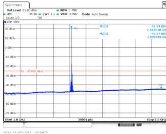
Band41_10MHz_QPSK_41190_1RB#0
