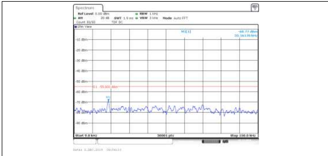
Band41_10MHz_QPSK_40690_1RB#0
