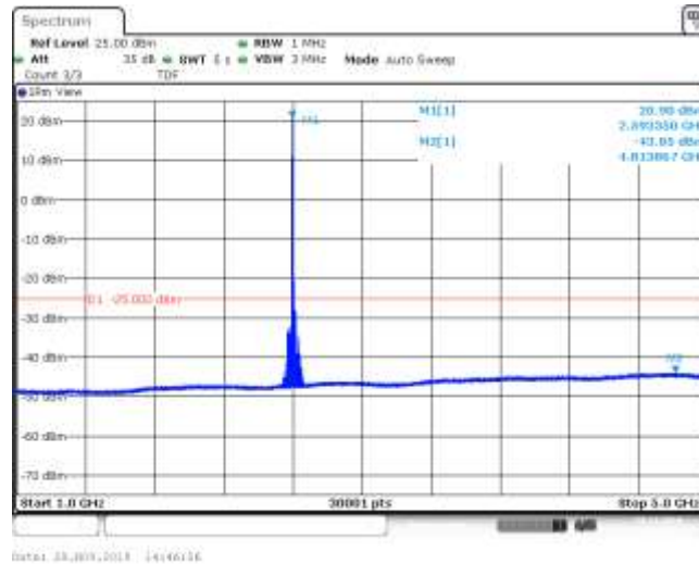
Band41_15MHz_QPSK_40690_1RB#0
