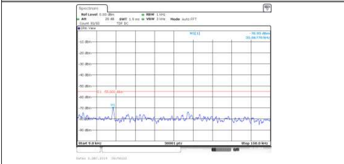
Band41_20MHz_QPSK_40690_1RB#0
