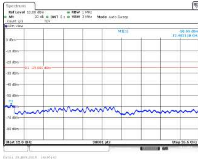
Band41_10MHz_QPSK_40290_1RB#0
