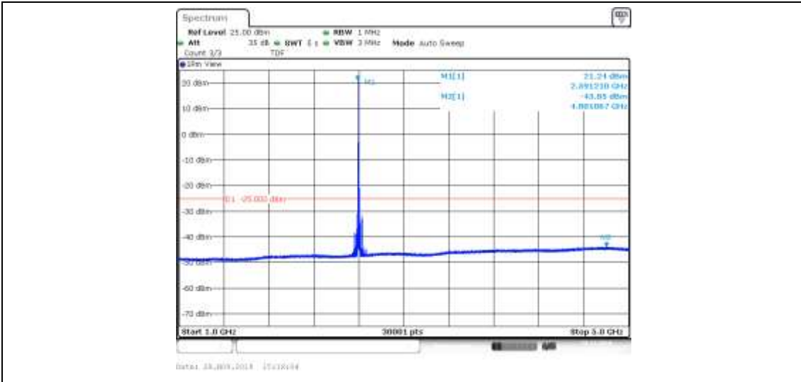
Band41_20MHz_QPSK_40690_1RB#0
