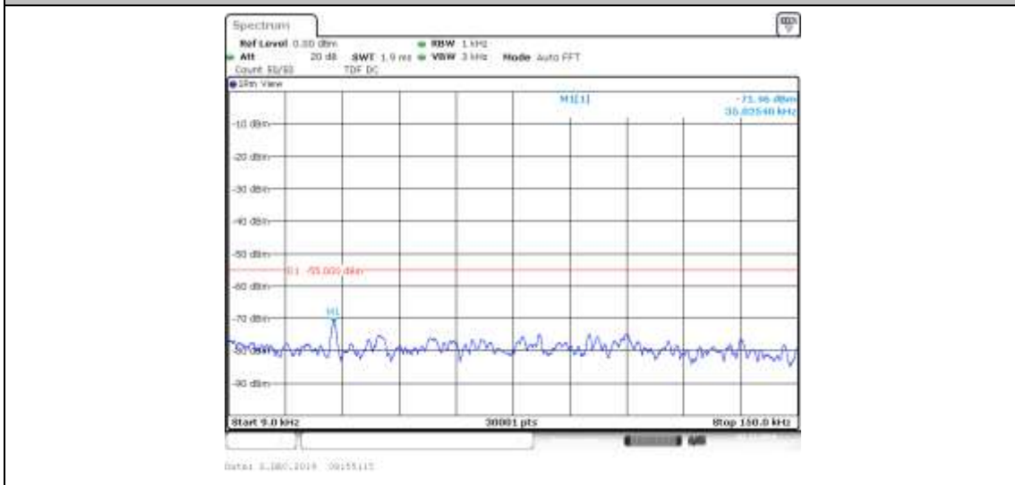
Band41_15MHz_QPSK_40690_1RB#0
