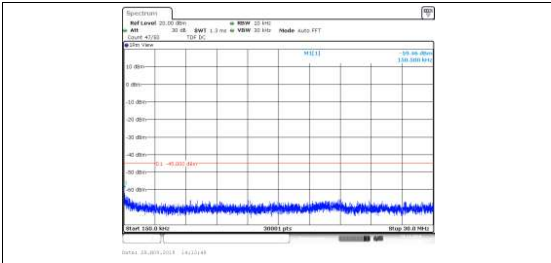
Band41_10MHz_QPSK_40290_1RB#0
