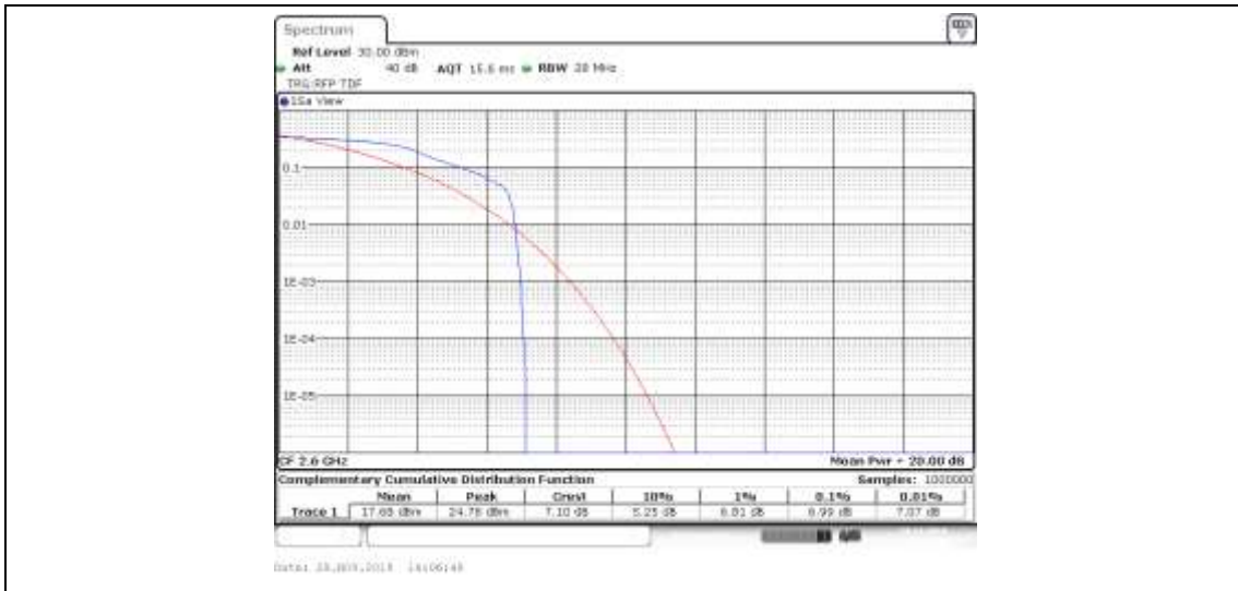
Band41_5MHz_QPSK_40690_25RB#0
