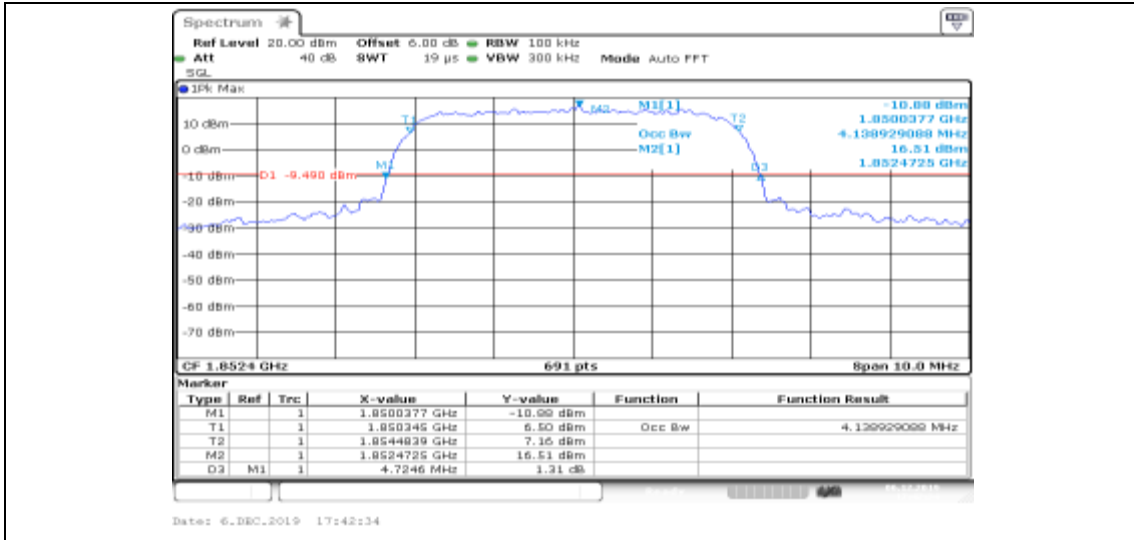
Band II-9262-HSUPA_Sub2
