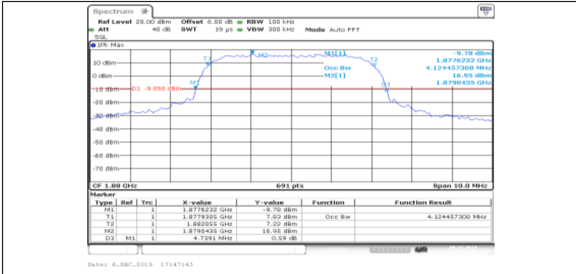
Band II-9400-HSUPA_Sub2
