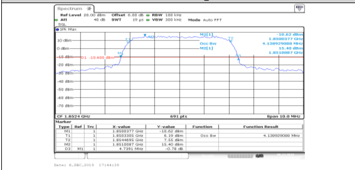
Band II-9262-HSUPA_Sub3
