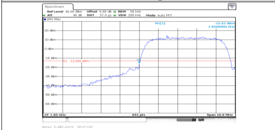
Band II-9262-HSUPA_Sub3
