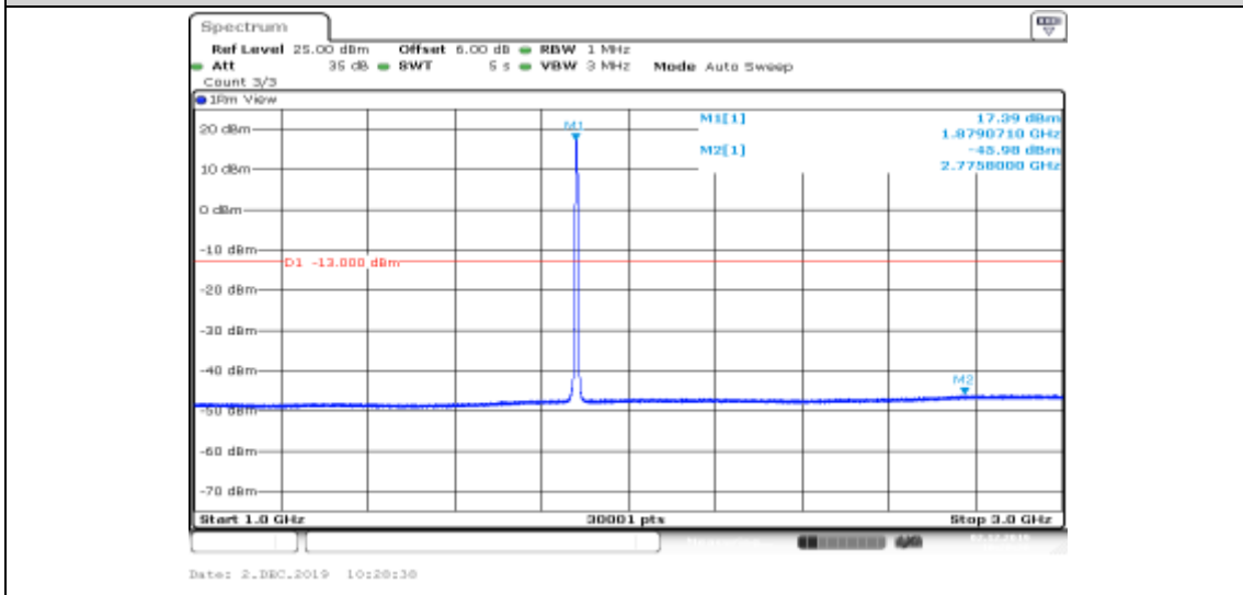
Band II-9400-1000~3000
