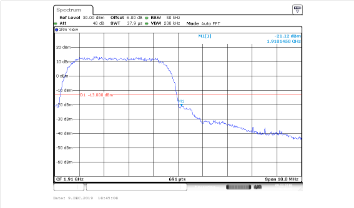
Band II-9538-HSUPA_Sub2
