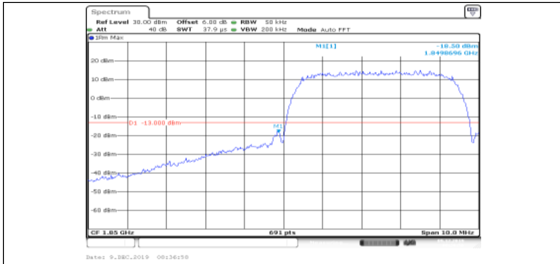
Band II-9262-HSUPA_Sub2
