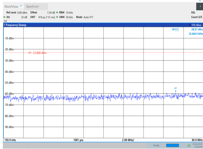
Band12-10MHz-QPSK-23060-1RB#0-Range2:0.15~30MHz
